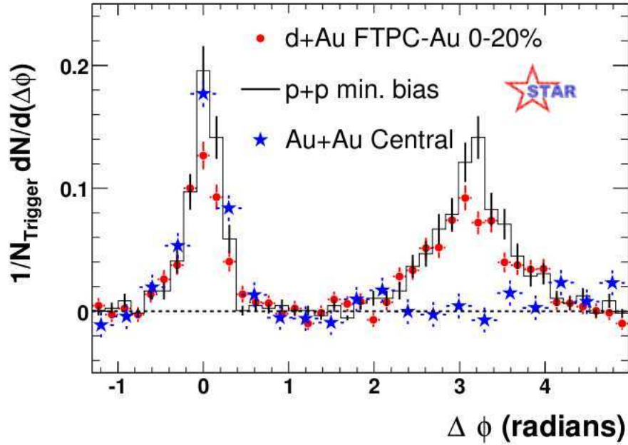
FIG. 1.11 – Correlations azimuthales des hadrons de haut p_t lors de collisions p - p , d - Au centrales et Au - Au centrales mesurées par l'expérience STAR [31].
