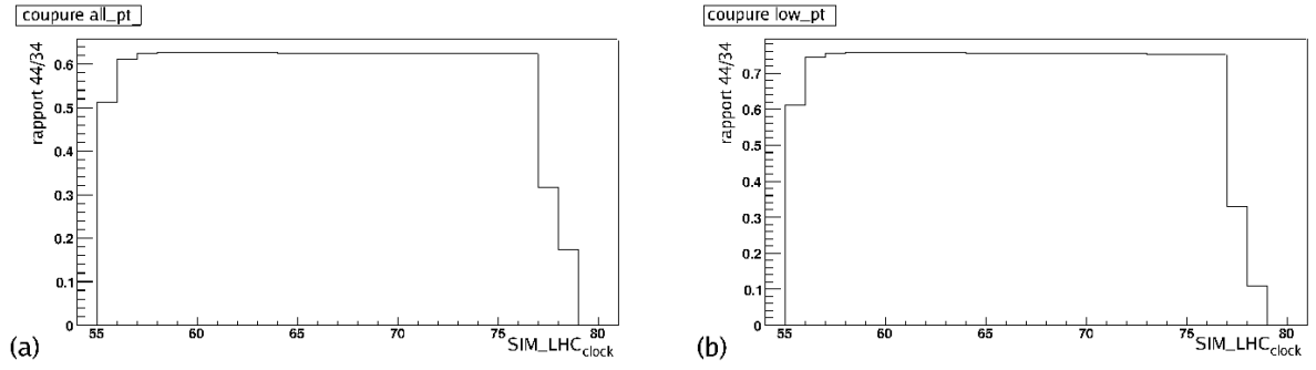
FIG. 4.12 – Simulation de collisions proton-proton minimum bias à \sqrt{s} = 14 TeV : rapport entre les coïncidences 4/4 et 3/4 All p_t (a) et Low p_t (b) en fonction de la variable SIM\_LHC_{clock} pour un résultat de référence n'incluant que les fluctuations dues au temps de vol.
