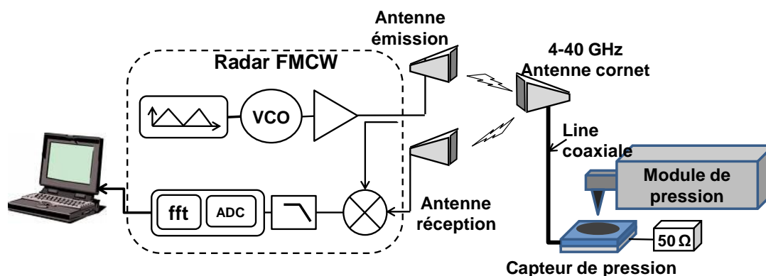
III-23 : Montage du système radar/capteur
