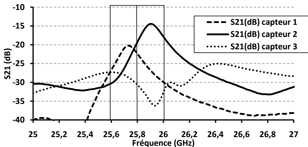
III-34 : Spectre en transmission des 3 capteurs
