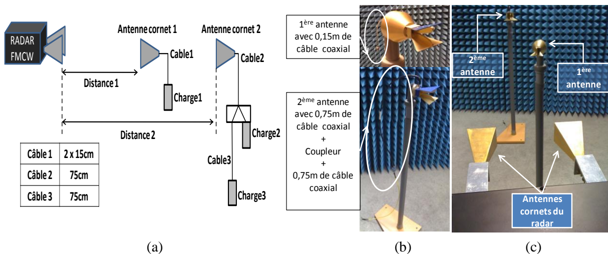
IV-1: (a) Montage expérimentale ; (b) antennes cornets n°1 et n°2 des capteurs (c) le Radar FMCW interrogeant les 2 antennes des capteurs à 1,5m et 3m de distances
