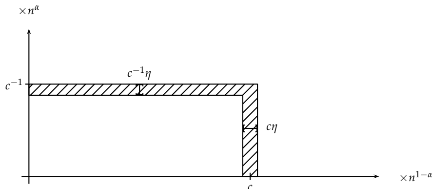
FIGURE 10.7 – Forme rectangle typique des diagrammes de Young renormalisés sous les mesures de Schur-Weyl de paramètre \alpha < 1/2 et c > 0 .
