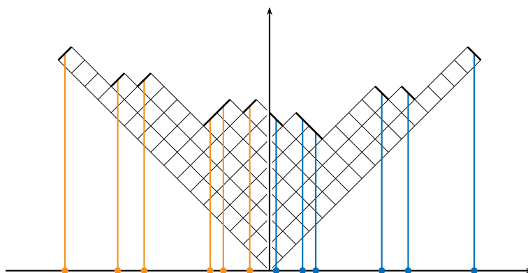
FIGURE 2.2 – Coordonnées de Frobenius d'un diagramme de Young.
