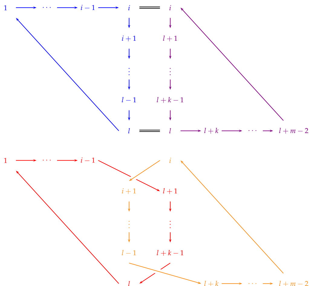
FIGURE 10.5 – Le produit de deux cycles C_l (en bleu) et C_m (en violet) s'intersectant en deux points d'écart (i, l - i) dans C_l et (k, m - k) dans C_m est égal au produit de deux cycles disjoints de longueurs respectives i + k - 1 (en rouge) et (l - i) + (m - k) - 1 (en orange).
