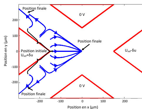
(d) Projection sur le plan ( xy ) des trajectoires d'une particule partant de plusieurs position initiales en appliquant une tension U = [100V, 0, 100V] .
