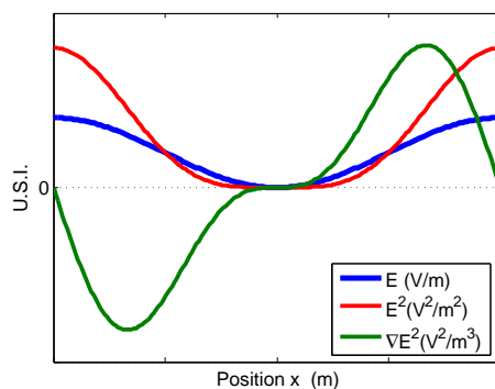
(a) Allure d'un champ électrique \vec{E} , de son carré \vec{E}^2 et du gradient du carré \nabla E^2 . Le champ est considéré uni-dimensionnel suivant l'axe x .
