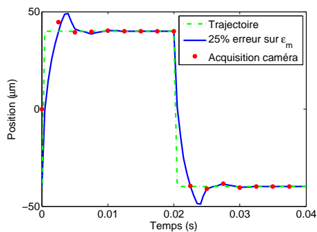
(a) Le suivi d'une trajectoire échelon d'amplitude de 40\mu m avec une perturbation de 25% sur la permittivité.
