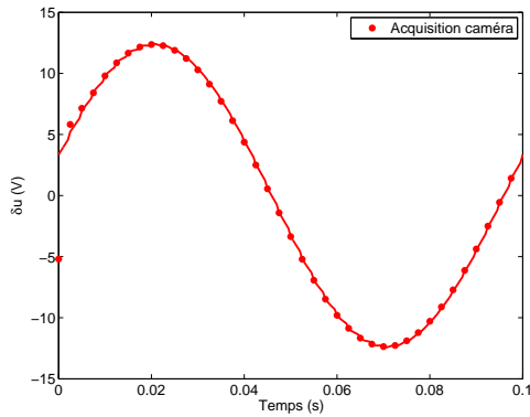
(c) Valeurs de la variable de commande \delta u calculées par le contrôleur GPC avec correction sur la consigne. On remarque l'absence des dents présentés dans l'exemple précédent.
