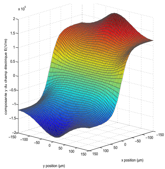
(b) Composante y de \vec{E} .
