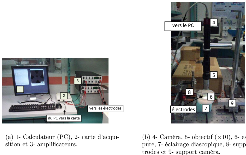
FIGURE 4.10 – Vue de l'ensemble des composants constituant le dispositif expérimental.
