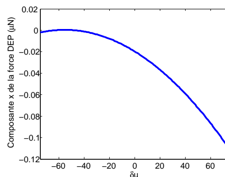
(b) Composante x de la force de diélectrophorèse calculée tout au point ( x = 0, y = 0, z = 50\mu\text{m} ) en appliquant une tension égale à U = [75 - \delta u, 0, 75 + \delta u] avec \delta u varie du -75V à 75V .
