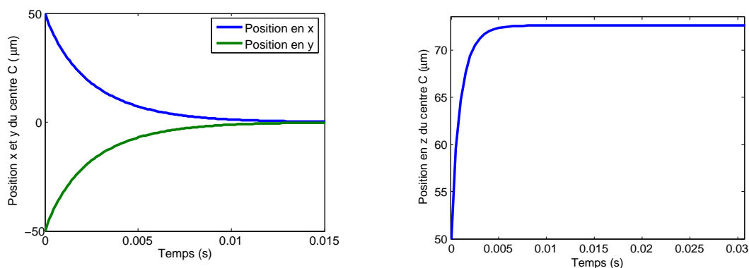
(a) Trajectoire suivant les directions x et y .
