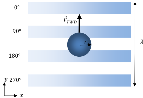
FIGURE 2.14 – Schéma montrant la force diélectrophorèse à onde progressive en appliquant des tensions électriques sinusoïdales déphasées.
