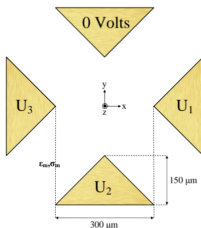
FIGURE 3.1 – Géométrie des électrodes utilisées dans les exemples de ce chapitre.
