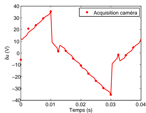
(b) La tension \delta u calculée pour le suivi d'une trajectoire échelon d'amplitude de 40\mu m avec une perturbation de 25% sur la permittivité.
