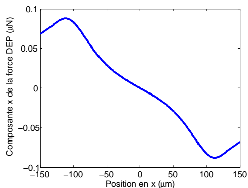
(a) Composante x de la force de diélectrophorèse calculée tout au long de l'axe ( y = 0, z = 50\mu\text{m} ) en appliquant une tension égale à U = [75V, 0, 75V] .
