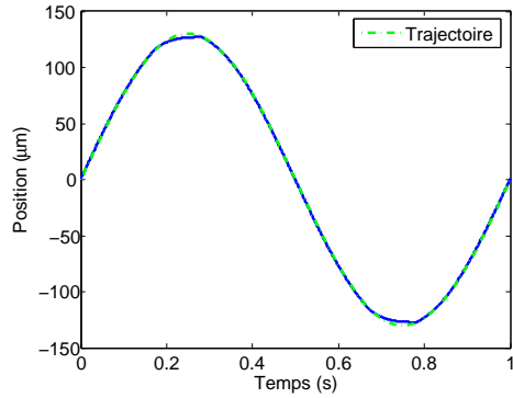
(a) Le suivi d'une trajectoire sinusoïdale de période égale à 1s et d'amplitude égale à 130\mu\text{m} . La commande se fait dans une zone fortement non-linéaire.
