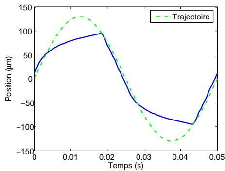
(a) Le suivi d'une trajectoire sinusoïdale de période égale à 50ms et d'amplitude égale à 130\mu\text{m} . La commande se fait dans une zone fortement non-linéaire.
