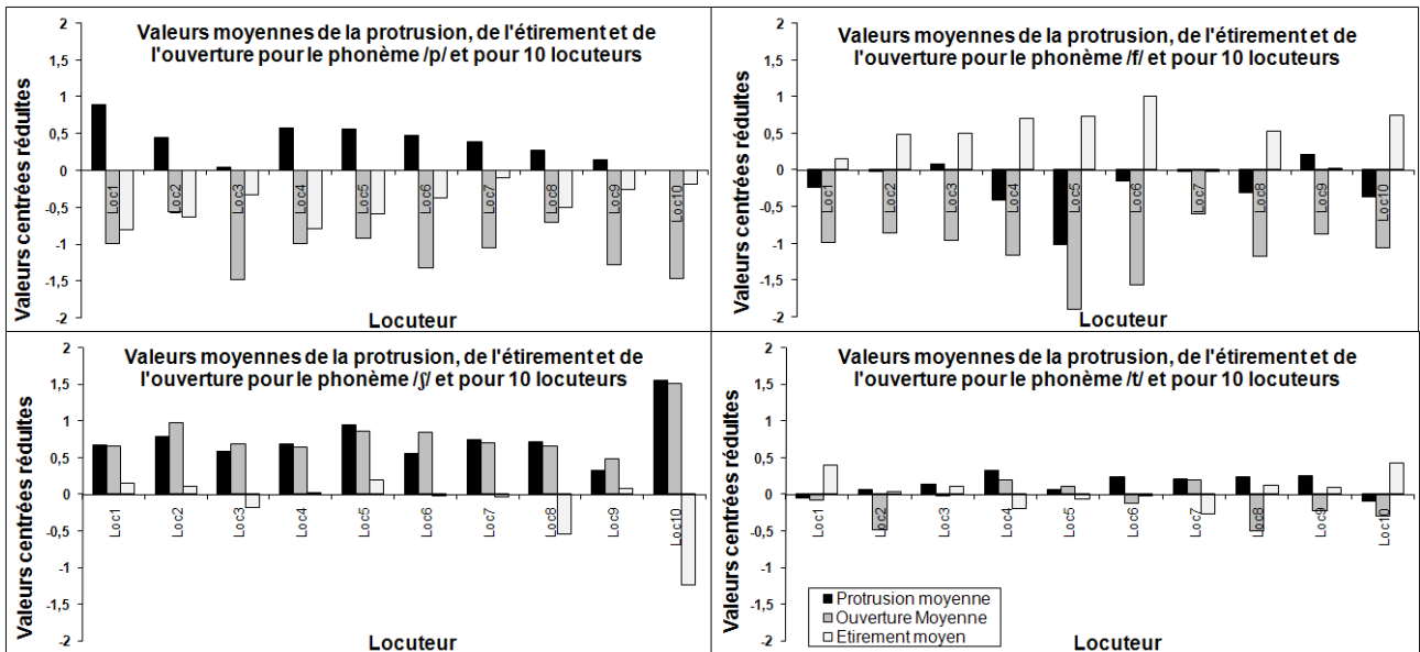
FIG. 4.16 – Moyennes centrées réduites des valeurs d’ouverture, de protrusion et d’étirement des consonnes pour chaque locuteur.
