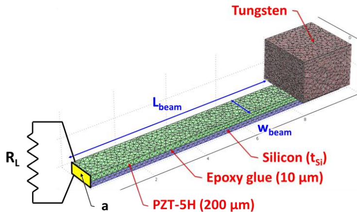
Fig. 23 - modèle éléments finis/SPICE
