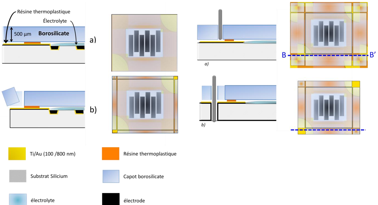
Fig. 64 – procédé d'encapsulation de l'électrolyte liquide : a) dépôt de résine photosensible et thermoplastique sur un substrat transparent (borosilicate ou silice fondue), b) découpe en 2 temps
