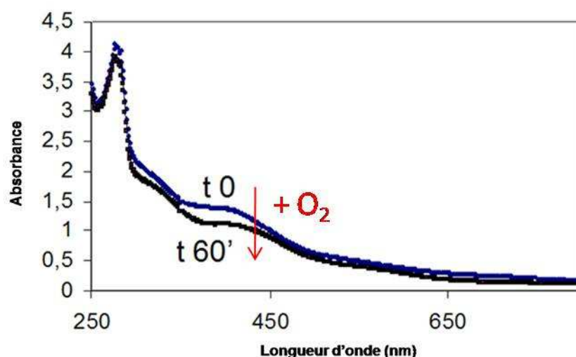
Figure 66 : Spectre UV-visible de la protéine NadA de T. maritima (250 \mu M) enregistré entre 250 et 800 nm. Le spectre en bleu est enregistré en absence d'oxygène. Le spectre en noir est enregistré après exposition de la protéine 60 min à l'oxygène.
