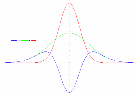
Figure 3.13 – Filtre différence de gaussiennes.
