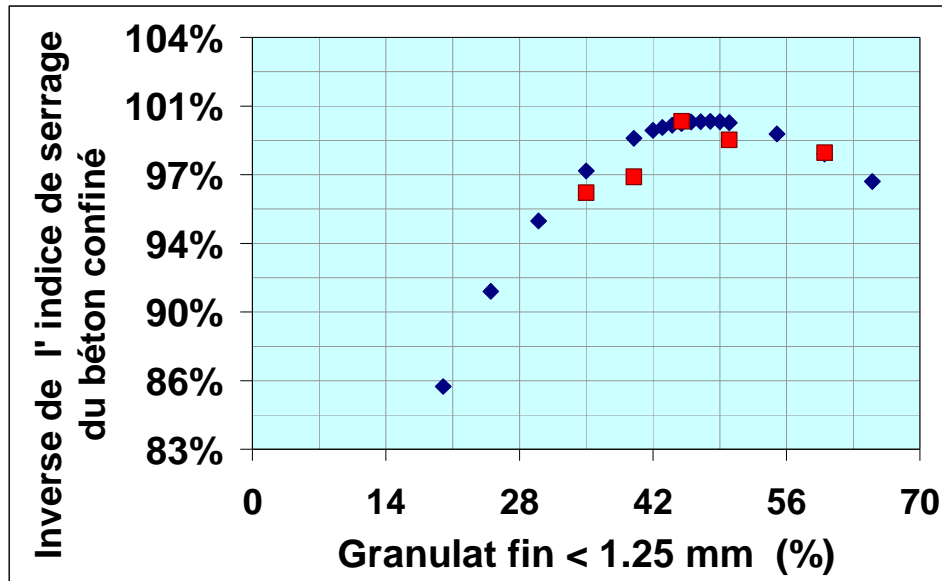
Figure 6.22- Optimisation granulairé modélisée en accord avec le MEC- BétonLab Pro 2 et résultats expérimentaux pour deux fractions de granulats. (Contraire de l'indice de serrage (%) vs. Résultats expérimentaux)
