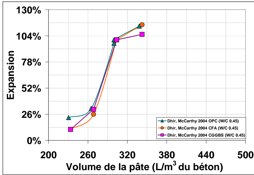
Figure 5.31- Expansion de poutrelles après une année d'exposition à une solution de 5% de Na_2SO_4 en fonction du volume de pâte et en termes relatifs quand la valeur de 300 L/m 3 de pâte correspond à une valeur de 100% [56].
