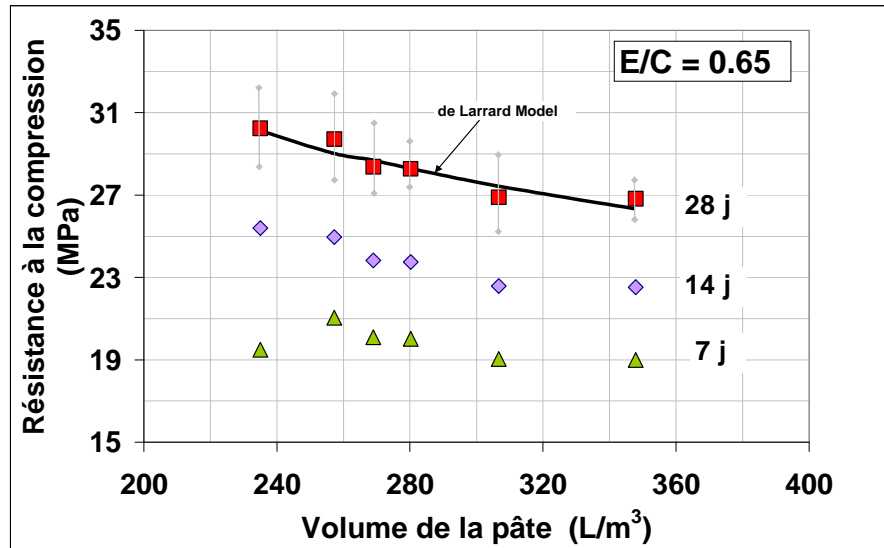
Figure 6.7- Volume de la pâte et résistance à la compression, avec le Modèle de Larrard. Série II.
