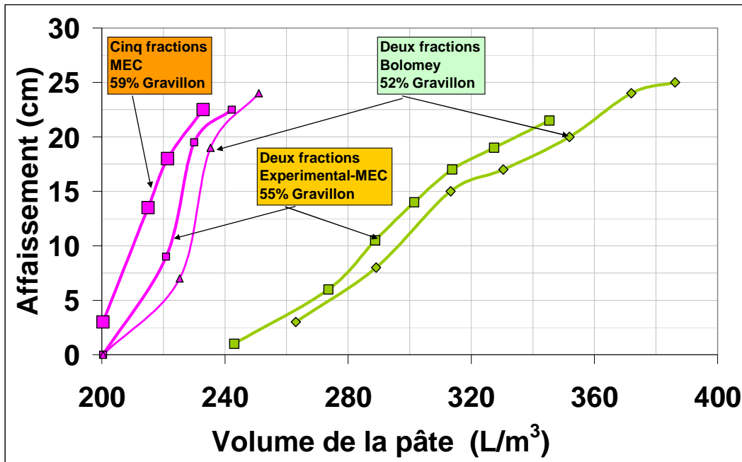
Figure 6.25-Effet du squelette granulaire sur la consommation de pâte.
