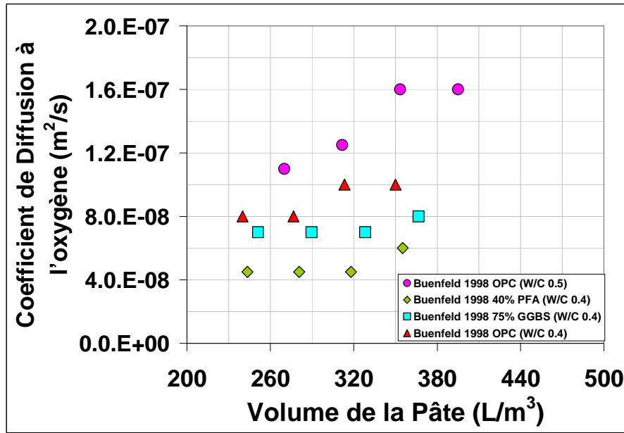
Figure 5.6 - Relation entre le coefficient de diffusion de l'oxygène et le volume de pâte d'après les résultats de Buenfeld et al.[8]
