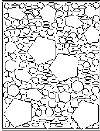
Fig 4.3 - Arrangement de granulat sans pâte.
