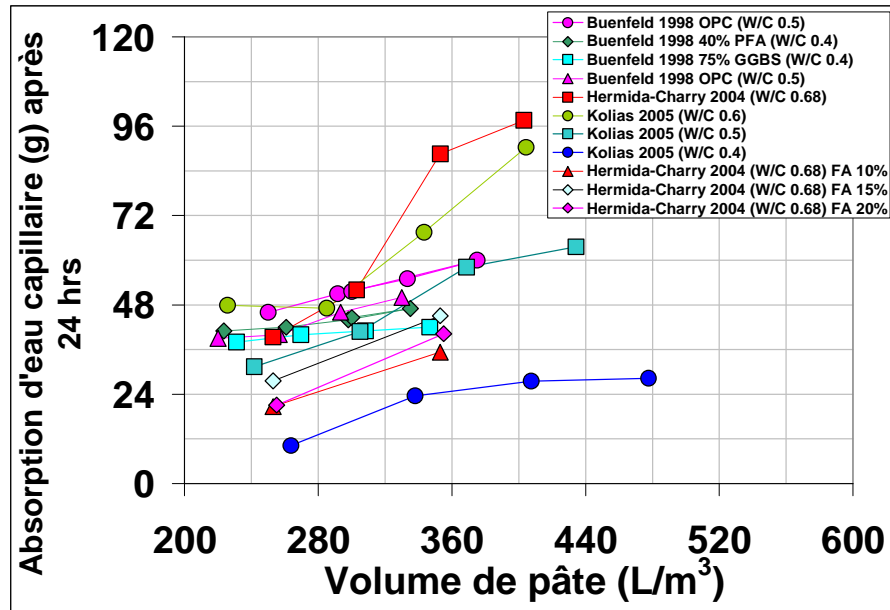
Figure 5.18-Relation entre la concentration de pâte ( V_c+V_w ) et l'absorption capillaire d'eau après 24 heures d'immersion de spécimens de béton cylindriques de diamètre 100 mm.
