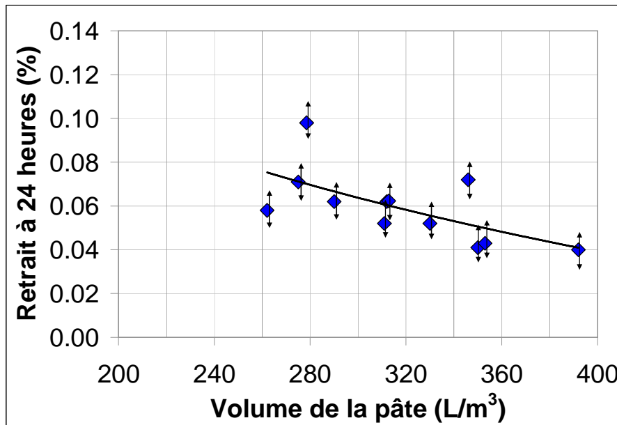
Figure 4.15- Volume de pâte vs retrait à 24 heures d'après Hermida et al [13] (E/C constant 0.46)
