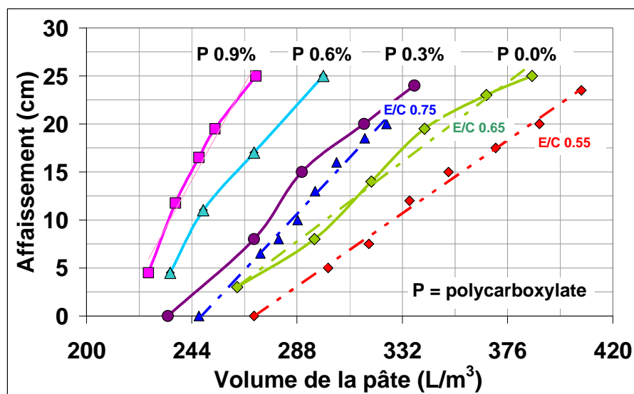
Figure 6.13- Consommation de pâtes avec différentes doses d'adjuvant et E/C constant de 0.65 avec la consommation de pâtes E/C =0.55 et E/C =0.75. (Superposition des Séries I et III)
