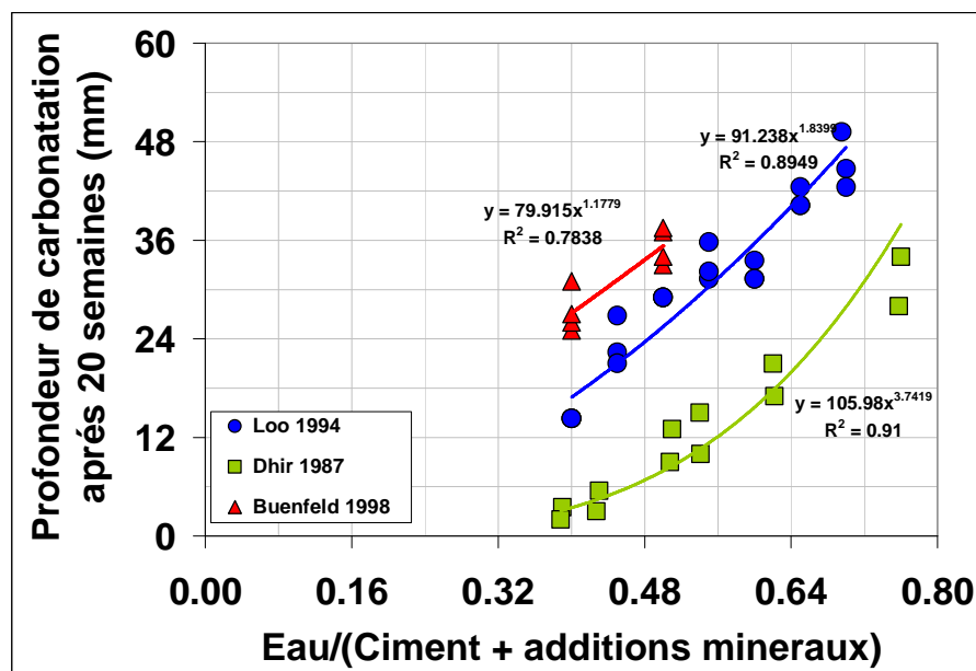
Figura 5.7- Rapport eau/ciment vs profondeur de carbonatation accélérée pour différents auteurs, obtenue sous des conditions similaires.
