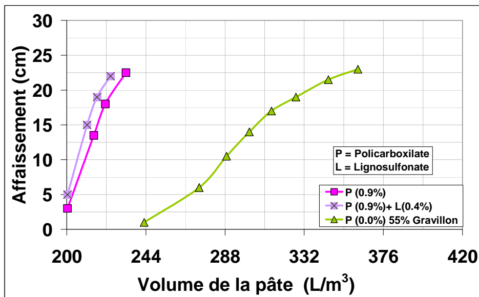
Figure 6.23- Consommation de pâte (E/C 0.65) pour un arrangement granulairé de 5 granulats optimisés en accord avec le modèle MEC et une dose d'adjuvant de 0.9% de polycarboxylate et 0.9% de polycarboxylate plus un plastifiant (Plastiment TM 5) à base de lignosulfonate. Série VIII
