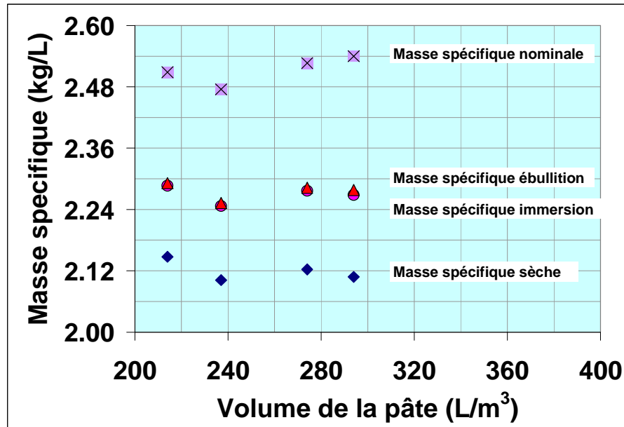
Figure 6.31- Volume de pâte ( E/C = 0.65 ) face à la masse spécifique sèche, nominal après immersion et ébullition. Série VIII.
