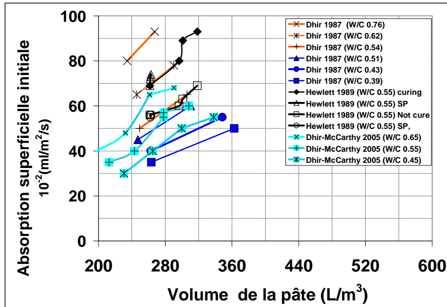
Figure 5.23-Volume de pâte vs Absorption Initiale de surface (ISAT-10) après 10 minutes d'absorption.
