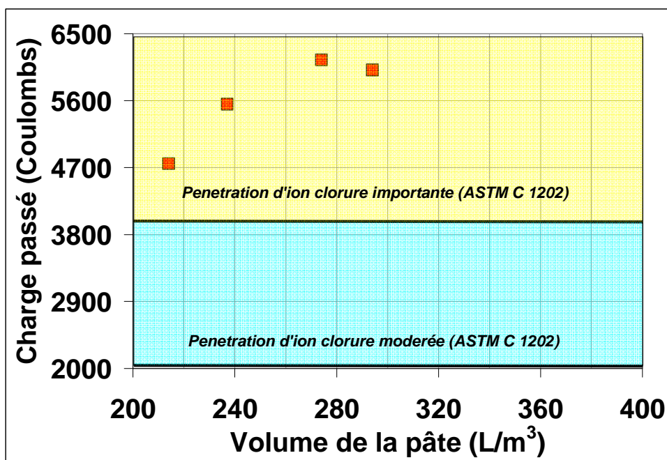
Figure 6.32- Volume de pâte ( E/C = 0.65 ) face à la charge électrique dans les bétons hautement optimisés. Série IX
