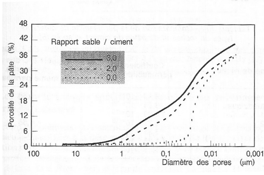
Figure 5.17 -Porosité de la pâte avec et sans sable d'après Feldman [150].
