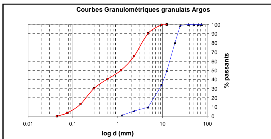
Figure 6.1- Distribution granulométrique des granulats Argos (Bogota) d'origine Tabio Tenjo.
