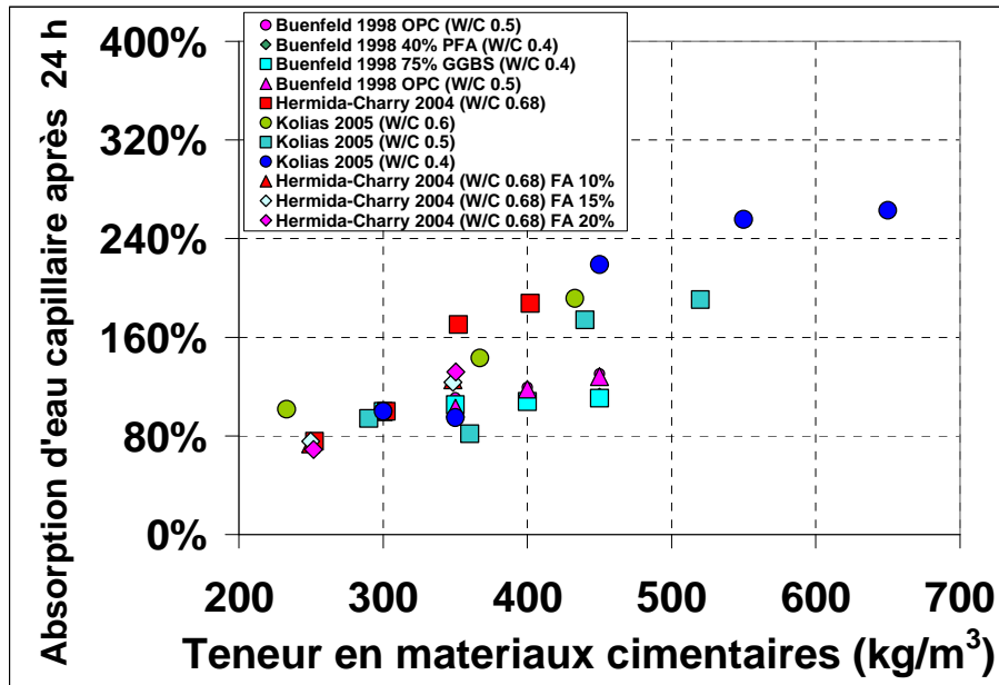
Figure 5.20-. Dosage de matériau cimentaire en fonction de l'absorption capillaire d'eau après 24 heures d'immersion de spécimens de béton cylindriques de diamètre 100 mm (%), où la valeur d'absorption capillaire pour 300 kg/m³ de ciment a été assumée à 100% de l'absorption.
