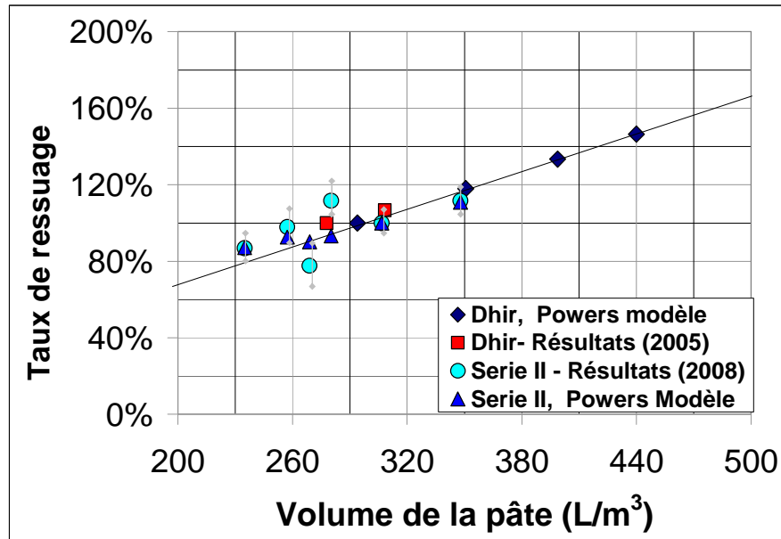
Figure 6.6- Relation entre le ressasse dans le temps et le volume de la pâte. Série II.
