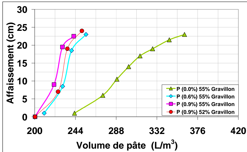
Figure 6.19- Consommation de pâte E/C = 0.65 pour différentes doses d'adjuvant et différents niveaux de maniabilité. Série VII. (Ciment CPR) T 20\text{ °C} - 65% HR avec l'optimum expérimental. P= Polycarboxylate
