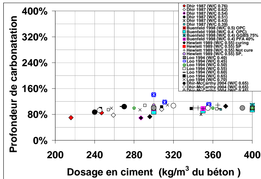
Figure 5.13 - Relation entre le contenu de ciment ( kg/m^3 ) et la profondeur de carbonatation accélérée et naturelle par différents auteurs.
