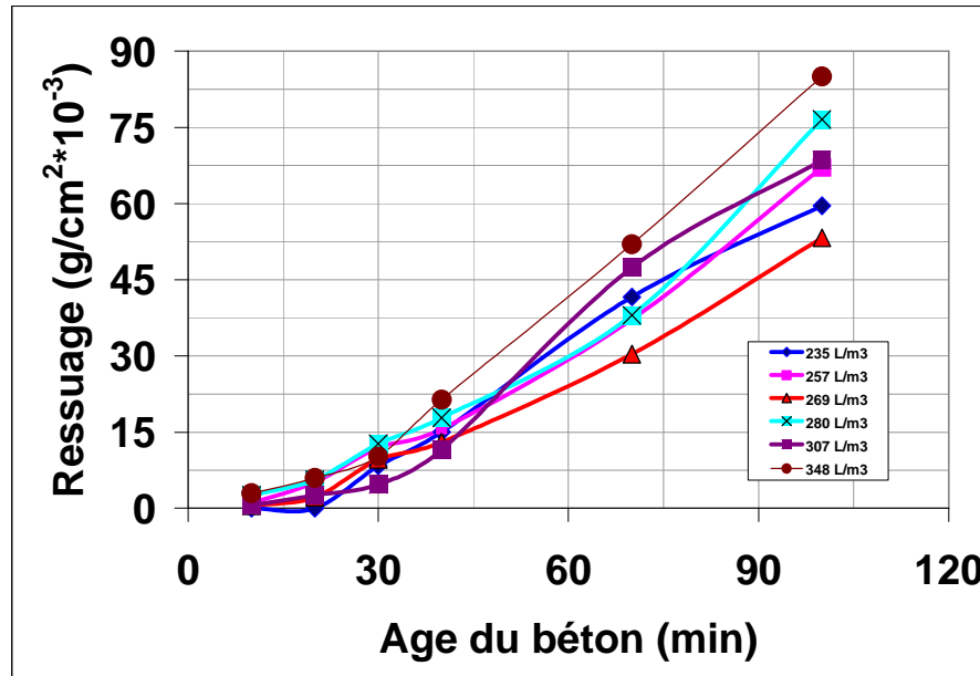
Figure 6.5- Relation entre le ressuage dans le temps et le volume de la pâte. Série II.
