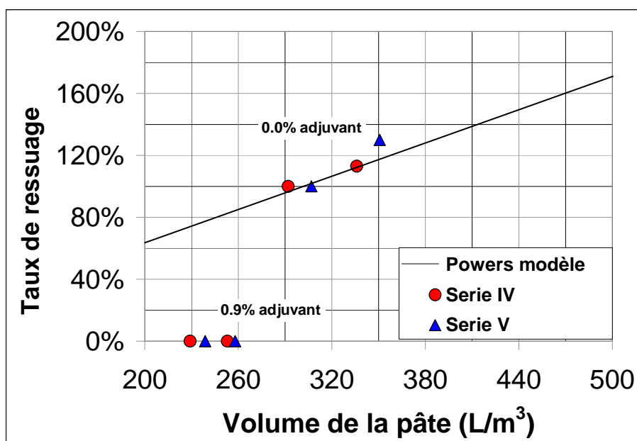
Figure 6.17- Ressuage cumulé ( g/cm^2 ) face au volume de pâte pour des bétons d'égal E/C et dosage d'adjuvant, en utilisant la méthode ASTM C 232 (Procédure A)
