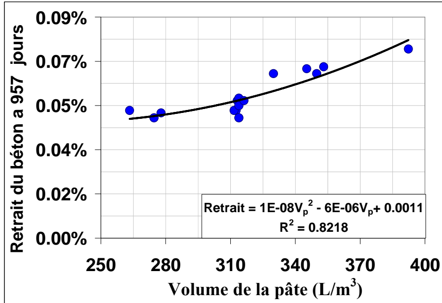
Figure 4.18- Retrait du béton à 957 jours (2.6 ans) vs. Volume de pâte/ m^3 [13]. ASTM C 157 échantillons 10*10*28.5 cm (HR 65\% \pm 5\% T 21 \text{ }^\circ\text{C} \pm 2 \text{ }^\circ\text{C} (E/C constant 0.46)).
