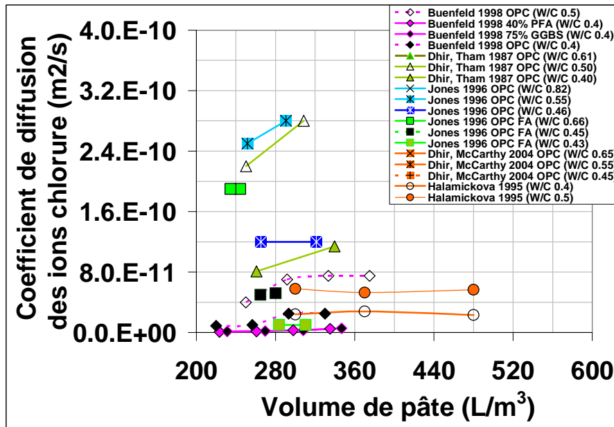
Figure 5.28-Coefficients de diffusion NaCl (m2/s) à partir de différents auteurs pour des séries de béton à égale qualité de pâte et différents contenus volumétriques de celle-ci.
