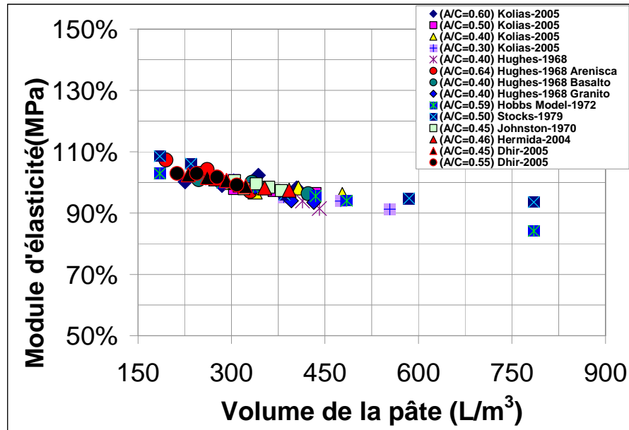
Figure 4.14- Volume de p te vs Module d' lasticit  d duit   partir des donn es exp rimentales de r sistance   la compression en employant le mod le ACI 318-08.
