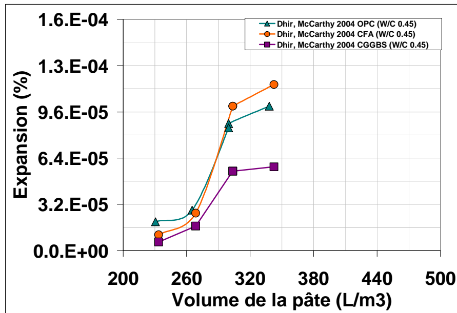
Figure 5.30-Expansion de poutrelles après une année d'exposition à une solution de 5% de \text{Na}_2\text{SO}_4 en fonction du volume de pâte [56].
