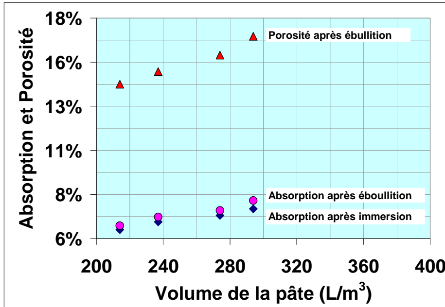
Figure 6.30- Volume de pâte ( E/C = 0.65 ) face à la porosité accessible à l'eau et, absorption en accord avec ASTM C642.
