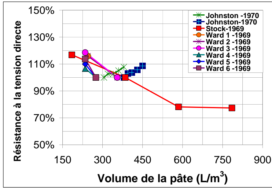
Figure 4.13- Relation entre le volume de pâte dans le béton et la Résistance à la traction directe selon différents auteurs [7,27,60].
