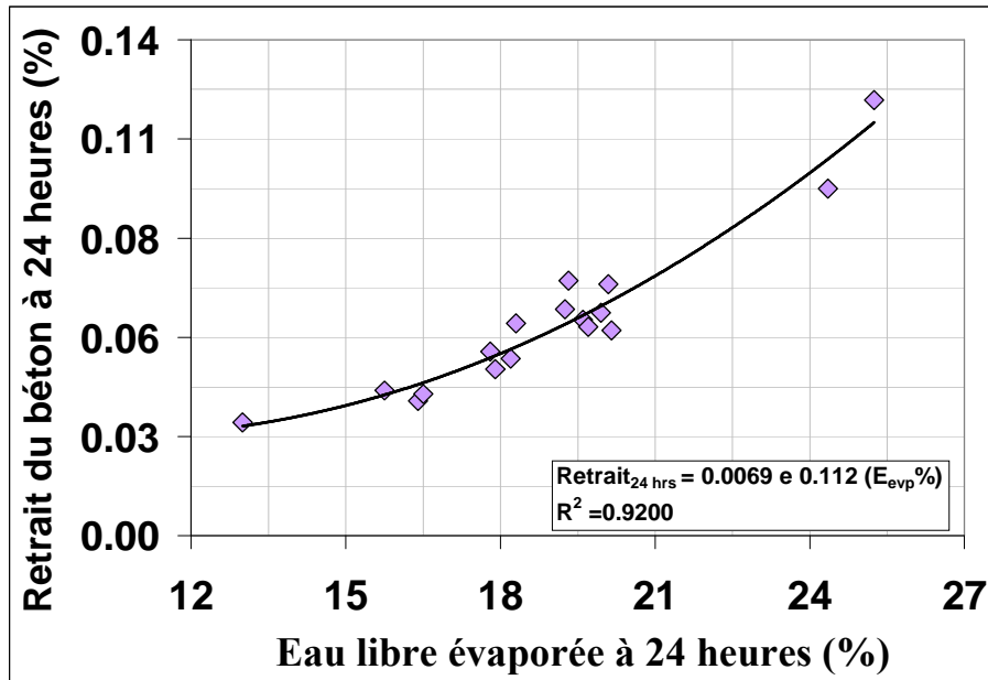
Figure 4.16- Pourcentage d'eau évaporée /eau libre vs Retrait aux 24 heures d' après Hermida et al. [13]
