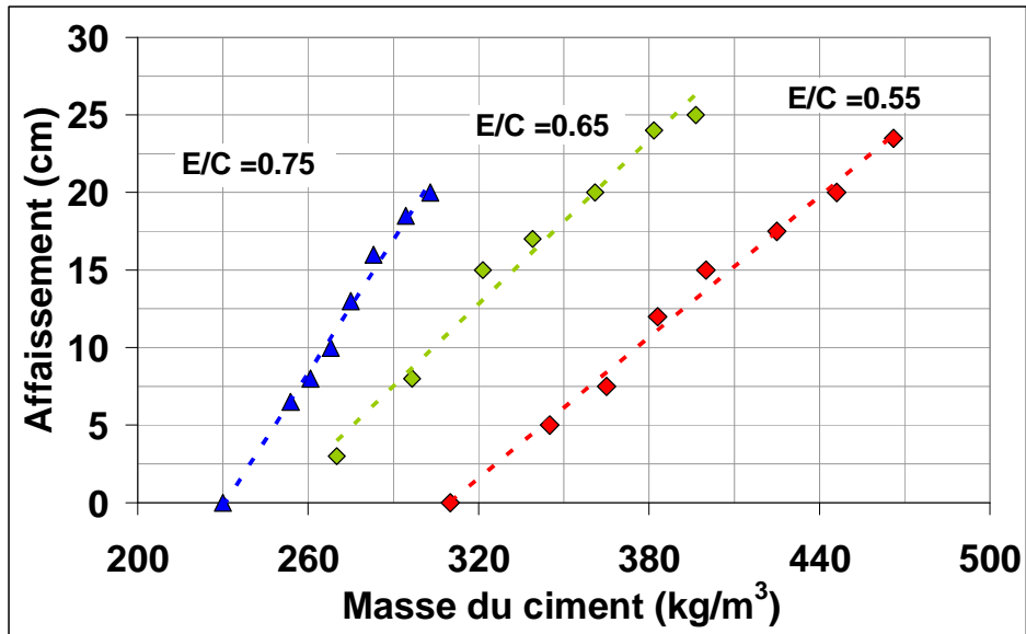
Figure 6.3- Consommation de ciment face à l'affaissement pour différentes qualités de pâte (E/C), Série I. Sensibilité de la concentration en ciment vs. Affaissement (ciment CPR) T 20^{\circ} C \pm 2^{\circ} C , HR 65\% \pm 5\%
