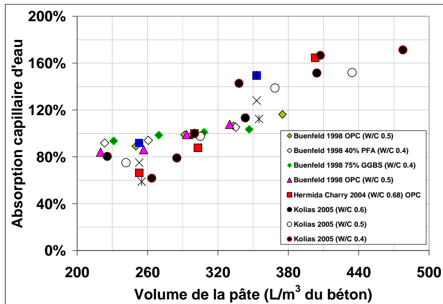
Figure 5.19- Concentration de pâte ( V_c+V_w ) fonction de l'absorption capillaire d'eau après 24 heures d'immersion de spécimens de béton cylindriques de diamètre 100 mm, où la valeur d'absorption capillaire pour 300 L a été prise comme un 100% d'absorption.
