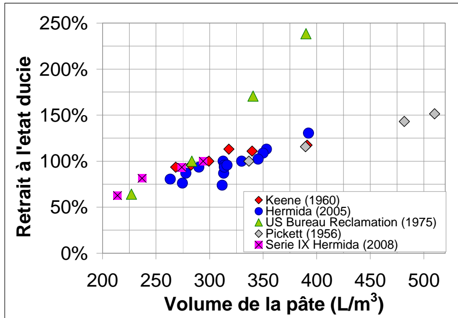
Figure 6.29- Retrait du béton à l'état durci face au volume de pâte, les résultats de la Série IX inclus. Valeurs exprimées en pourcentage du retrait obtenu par un béton avec 300 L/m 3 de pâte.
