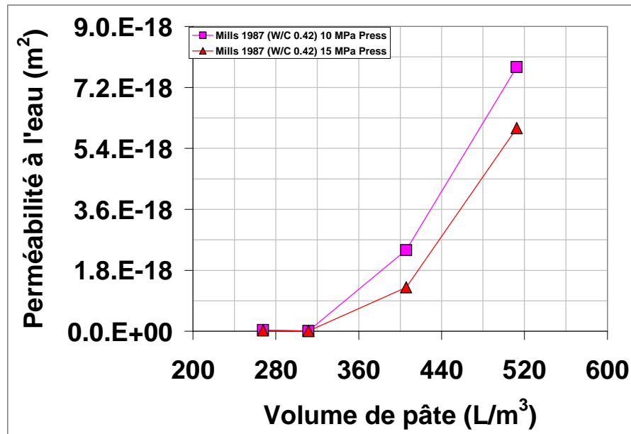
Figure 5.15- Perméabilité intrinsèque de bétons pour une qualité constante de pâte (E/C= 0.42) et un volume de granulats variable. La pression d'eau est de 1.38MPa pour deux pressions latérales de 10MPa et 15MPa.
