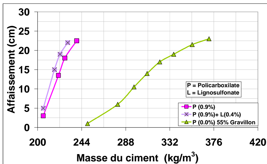
Figure 6.24-Consommation de ciment (E/C 0.65) pour un arrangement granulaire de 5 granulats optimisés en accord avec le modèle MEC et une dose d'adjuvant de 0.9% de polycarboxylate et 0.9% de polycarboxylate plus un plastifiant à base de lignosulfonate.
