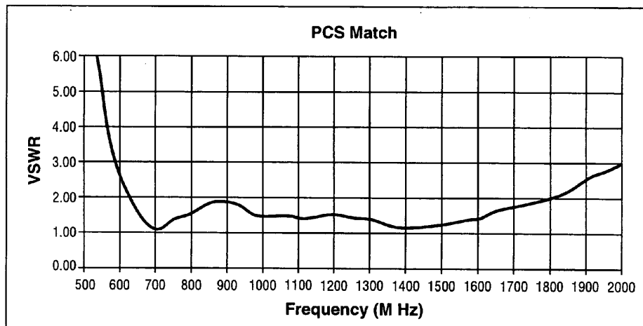
FIGURE 2.37 – ROS du car-antenna excité par une antenne de type disc-cône
