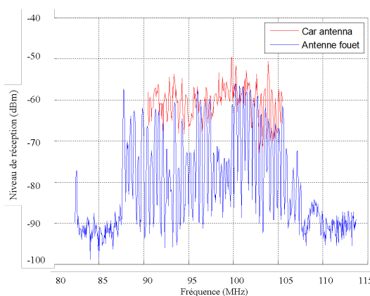
FIGURE 5.11 – Enregistrement de spectre du car-antenna amplifié en mode diversité et de celui du fouet sur le site de PSA-Velizy ( 48^{\circ}45'59.370''N ; 2^{\circ}12'57.300''E )
