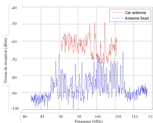
FIGURE 5.12 – Enregistrement de spectre du car-antenna amplifié en mode diversité et de celui du fouet sur la descente de Bièvres ( 48^{\circ}45'17.742''N ; 2^{\circ}12'53.676''E )
