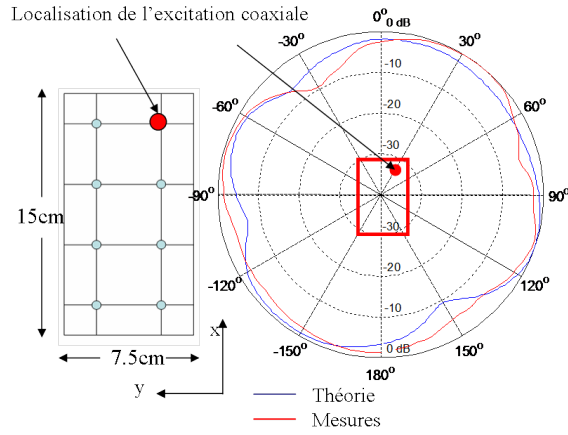
FIGURE 3.31 – Comparaison des diagrammes de rayonnement ( E_{\theta} ) normalisés théoriques et mesurés en azimut ( \theta = 90^{\circ} ) du parallélépipède à 2GHz ; excitation au point P1 ( x = 131.5mm ; y = 56.25mm )
