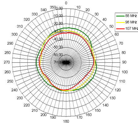
FIGURE 4.14 – Diagrammes de rayonnement ( E_{\theta} ) mesurés du car-antenna en azimut ( \theta=90^{\circ} ) pour les fréquences 88MHz, 98MHz, 107MHz; branchement sur la boucle d'attache de la ceinture de sécurité
