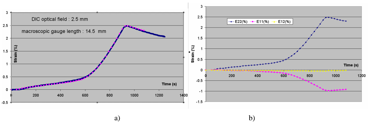
a) b) Figure 60 : Zirconium grade 702 soumis à un essai de traction à la température ambiante. a) Evolution de la déformation axiale au cours du temps pour différentes base de mesure. b) Evolution des composantes 11, 22, et 12 (base de mesure millimétrique)
