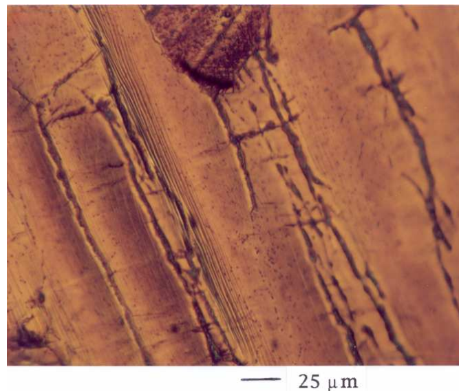
Figure 14a) Mise en évidence au moyen de la technique d'oxydation ménagée d'un gradient de composition chimique en oxygène au sein des lamelles de zirconium. Localisation du glissement prismatique le long des joints de lattes dans les zones appauvries en éléments d'addition alphas. [Crépin, 95]
