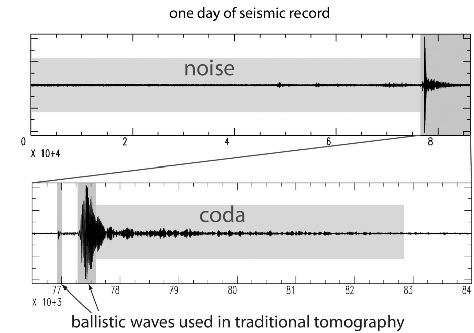
FIG. 1.2 – Exemple d’enregistrement en continu durant une journée incluant un séisme de grande magnitude. 95 % environ de l’enregistrement sont constitués de bruit, 4 % de la coda. Les ondes balistiques utilisées en tomographie traditionnelle ne constituent que 1 % du signal.
