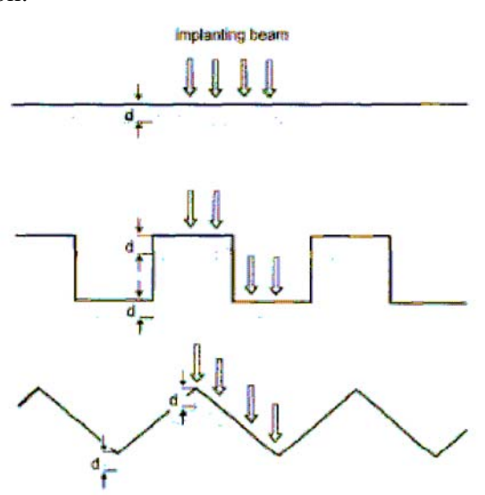
Figure C-1 : Profondeur d'implantation à incidence normale [BEHRISCH].
