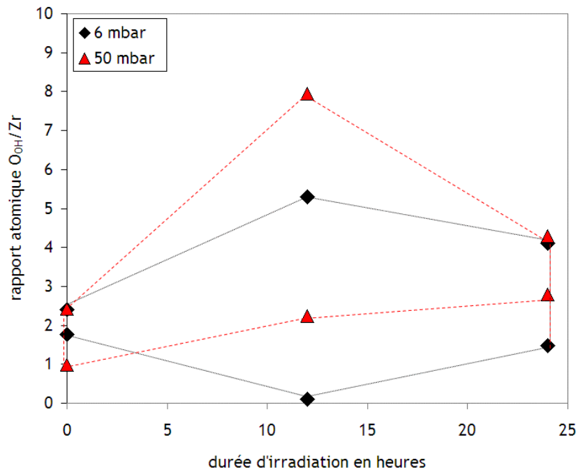
Figure IV-17 : Rapport atomique O_{OH}/Zr en fonction du temps de contact pour les essais réalisés à 6 et 50 mbar
