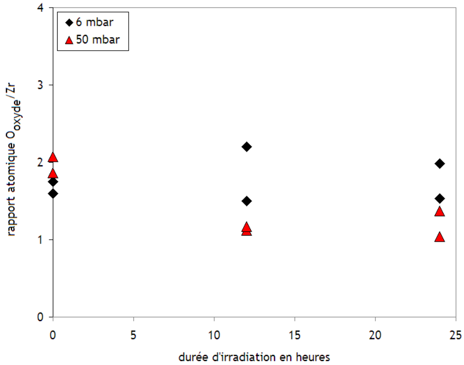
Figure IV-16 : Rapport atomique O_{oxyde}/Zr en fonction du temps de contact pour les essais réalisés à 6 et 50 mbar
