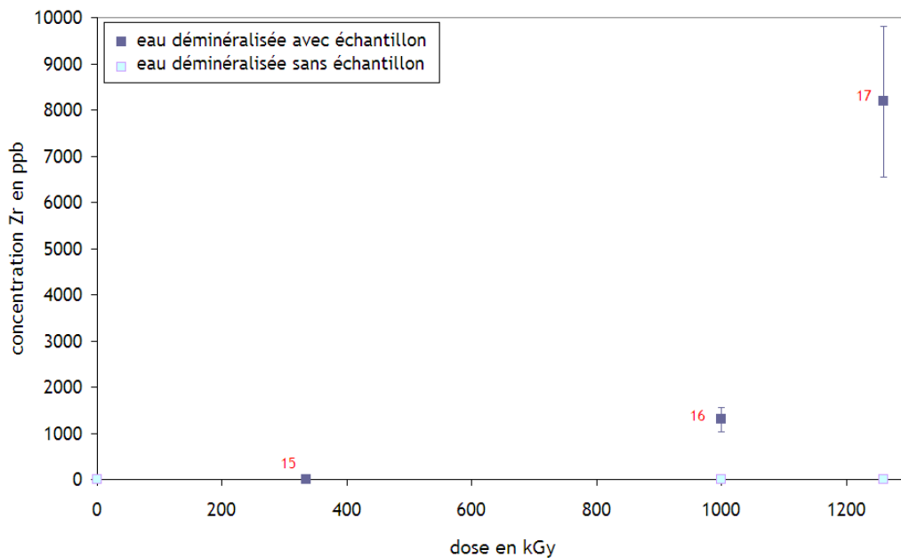
Figure V-11 : Concentration en ppb massique en zirconium en fonction de la dose délivrée dans l'eau pour les échantillons en contact avec l'eau déminéralisée irradiée. La limite de détection est de 1 ppb.
