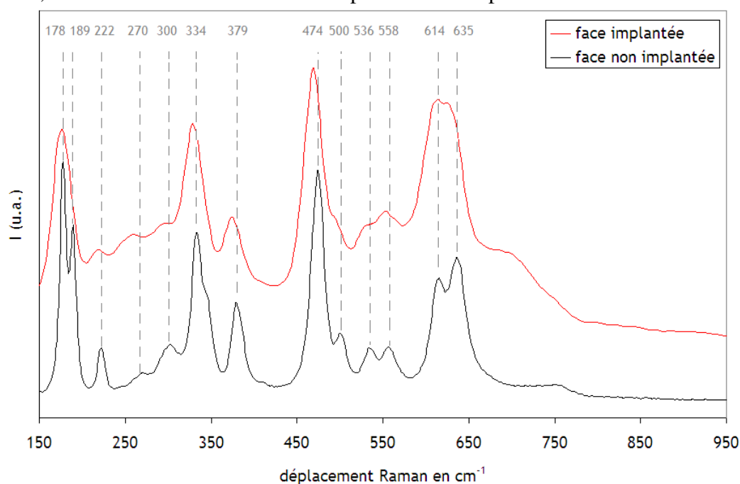
Figure III-7 : Spectres Raman obtenus sur le même échantillon après oxydation, seule une face est implantée en europium.
