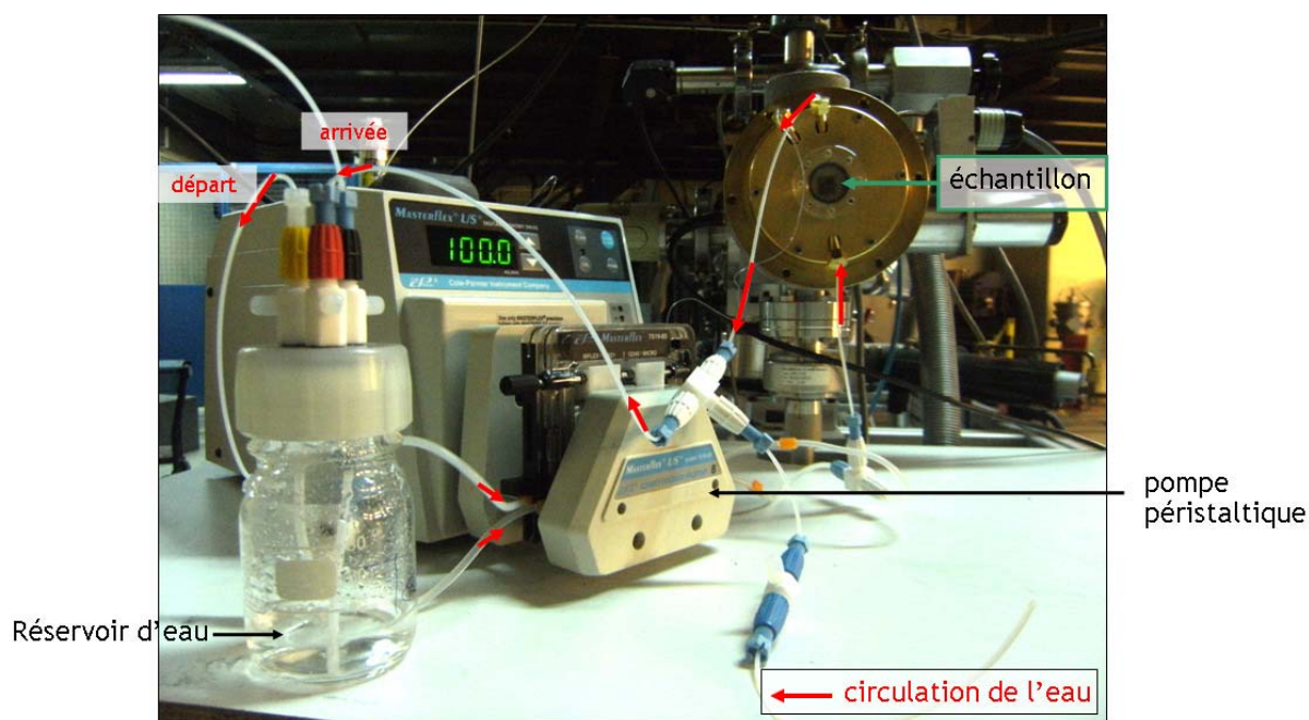
Figure III-26 : Photo de la cellule d'irradiation zirconium/eau/proton
