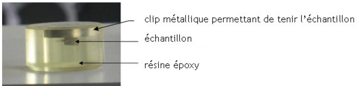
Figure III-4 : Echantillon enrobé dans une résine époxy
