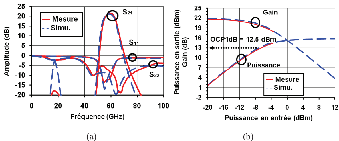
Figure 3 : Paramètres S (a), gain en puissance et puissance en sortie (b) de l'amplificateur de puissance
