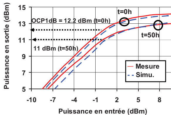
Figure 13 : Comparaison entre la mesure et la simulation de la puissance en sortie avant et après un stress de 1,78 V et P_e = 0 \text{ dBm} pendant 50 h
