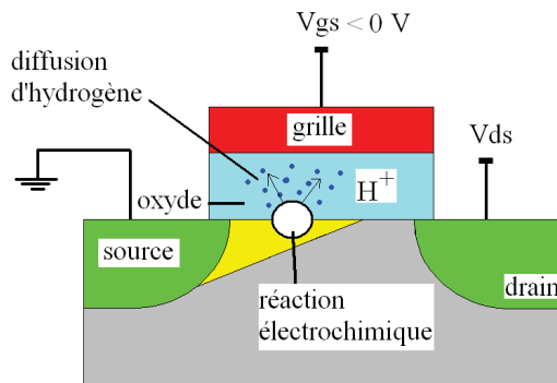
Figure 15 : Principe du mécanisme réaction-diffusion dans une dégradation de type NBTI
