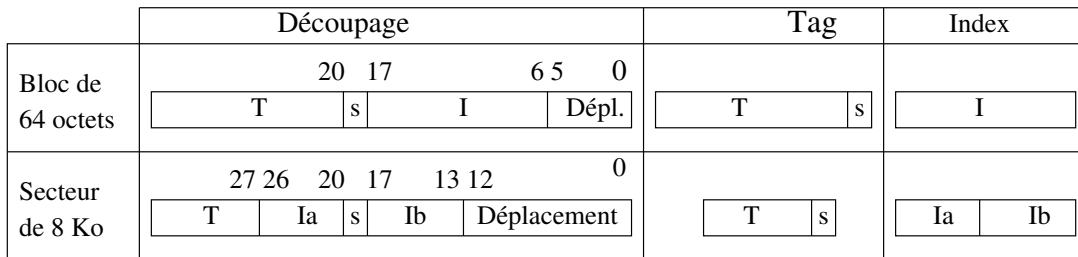
FIGURE 3.13 – Exemple du format d'adresse avec un cache de 1 Mo, 8 voies, des blocs de 64 octets et des secteurs de 8 Ko.
