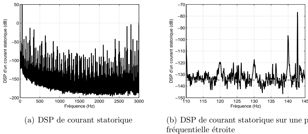
FIG. 4.6 – Densité spectrale de puissance d'un courant statorique
