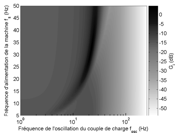
FIG. 3.26 – Gain G_i pour une fréquence statorique 5Hz \leq f_s \leq 50Hz
