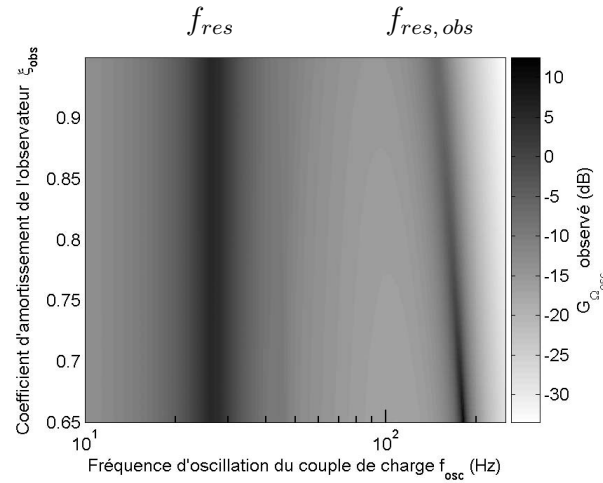
FIG. 5.15 – Gain G_{\hat{\Omega}_{osc}} pour un facteur d'amortissement de l'observateur 0.65 \leq \xi_{obs} \leq 0.95 , un gain d'observation G_{obs} = 10 et une fréquence d'alimentation f_s = 50Hz
