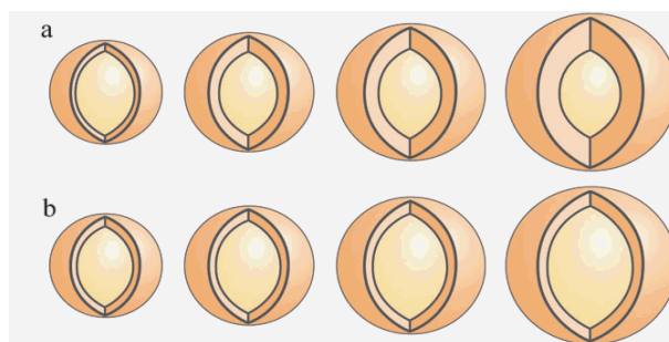
FIG. 2.6 – Mélanges d'aérosols en core-shell caractérisés par : (a) Un noyau de taille constante et une enveloppe d'épaisseur variable et (b) un noyau de taille variable et une enveloppe d'épaisseur constante, (source Lang-Yona et al. (2009)).
