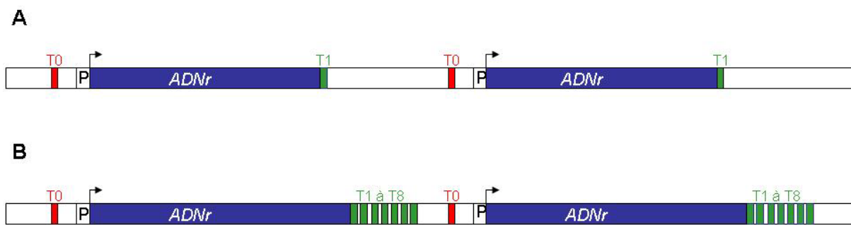
Figure 27 : Localisation des éléments terminateurs au sein de l'unité d'ADNr. (A) Représentation schématique de deux unités successives d'ADNr ribosomique de S. cerevisiae . La séquence transcrite par l'ARN polymérase I est indiquée par une boîte bleue. Le promoteur est noté par un « P ». L'élément de pause T1 est indiqué en vert, le terminateur proximal T0 est indiqué en rouge. (B) Représentation schématique de deux unités successives d'ADNr ribosomique de mammifère. La séquence transcrite par l'ARN polymérase I est indiquée par une boîte bleue. Le promoteur est schématisé par un « P ». Les éléments de pause T1 à T8 sont indiqués en vert, le terminateur proximal T0 est indiqué en rouge.
