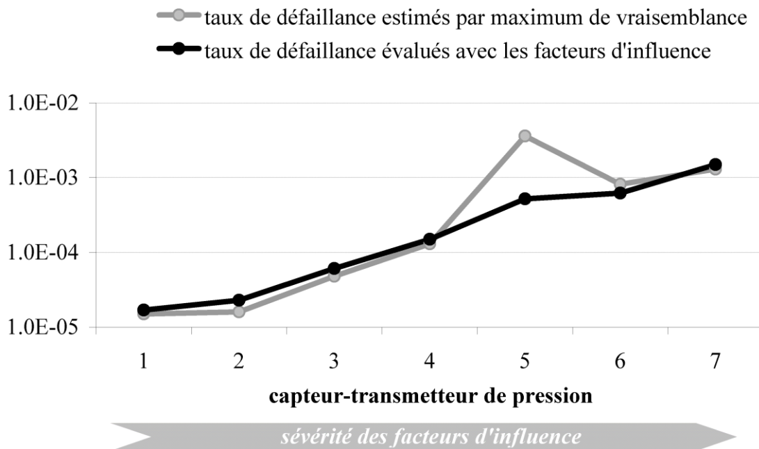
Figure II.2.7. Résultats des évaluations des taux de défaillance avec les facteurs d'influence, et des estimations par maximum de vraisemblance, pour les capteurs-transmetteurs de pression données dans le Tableau II.2.3
