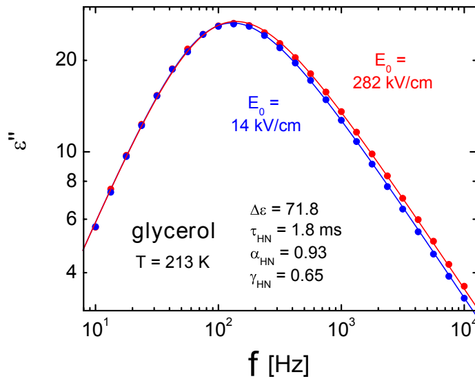
FIGURE 1.16 – Mesure de \epsilon'' en fonction de la fréquence f sur le glycérol à 213 K pour deux champs : E_0 = 14 kV/cm (en bleu) et E_0 = 282 kV/cm (en rouge). Les lignes pleines sont en bleu l'ajustement d'une loi d'Havriliak-Negami (voir partie 3.1.1.2) et en rouge la prédiction de l'équation 1.14 [30].
