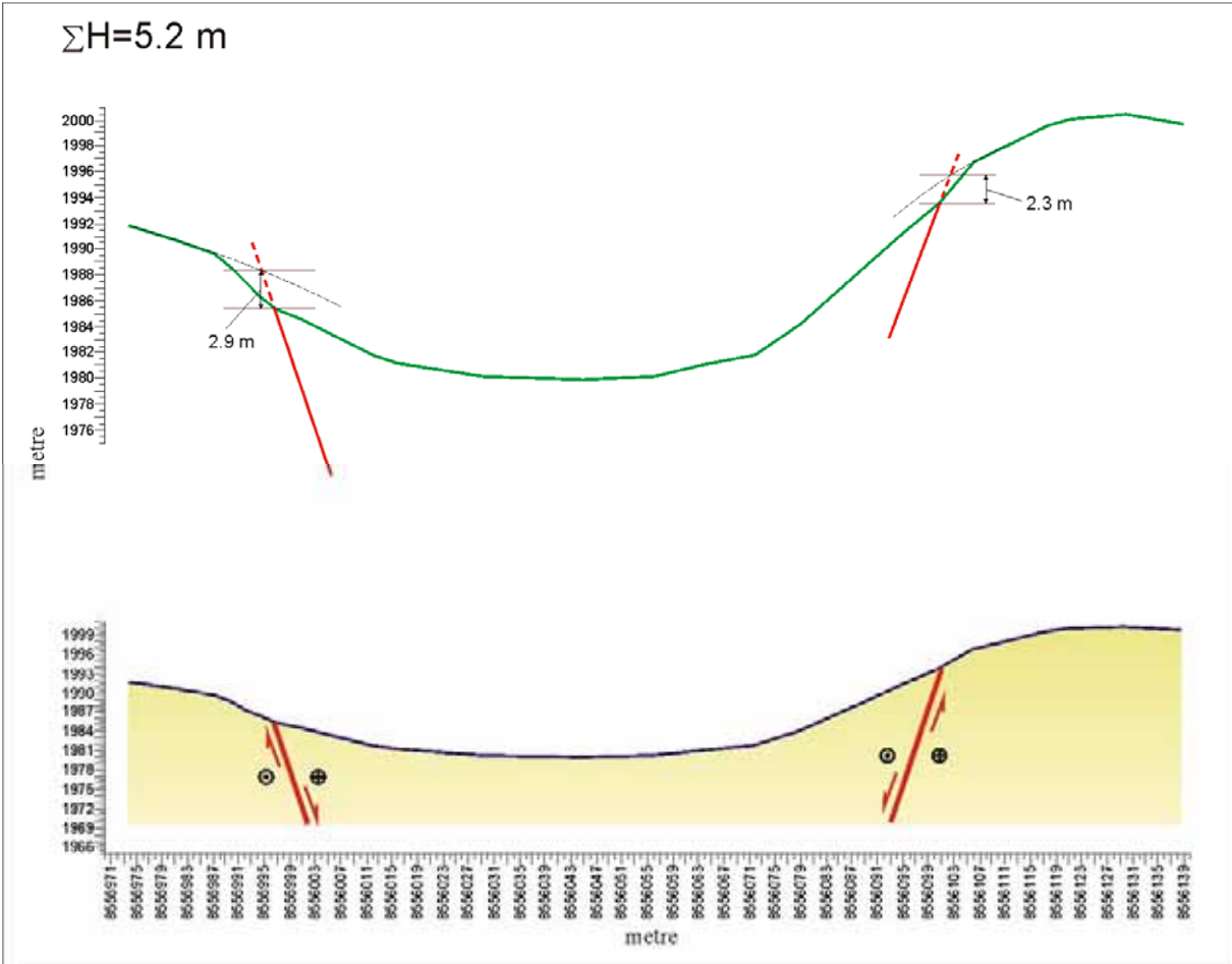
Profil 19-19'
