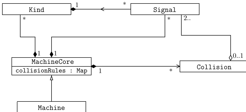
FIG. A.4 – Classes pour les machines.
