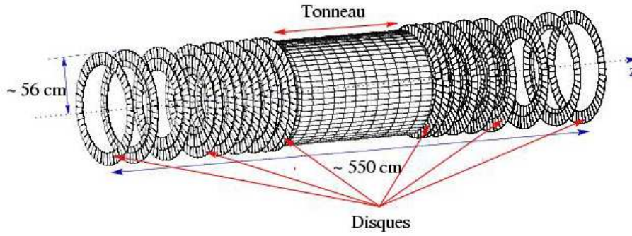
FIG. 2.7 – Shéma du détecteur SCT.
