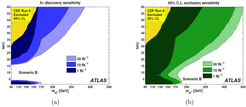
FIG. 5.7 – Sensibilité estimée en termes de contours de découvertes à 5 \sigma (a) et de contours d'exclusion à 95% de niveau de confiance (b), de la recherche du boson de Higgs chargé dans ATLAS en combinant tous les modes de recherche qui ont été étudiés dans [23].
