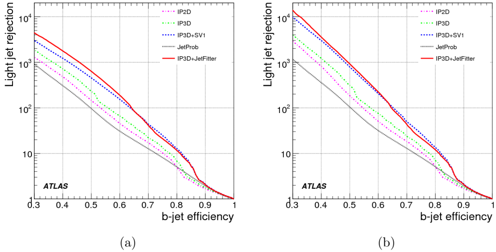
FIG. 3.11 – Rejet des jets légers (a) et des jets légers purifiés (b) obtenu sur des événements t\bar{t} pour différents algorithmes d’étiquetage en fonction de l’efficacité d’étiquetage.
