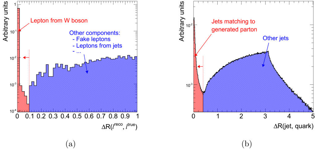
FIG. 6.2 – Distribution de la distance \Delta R entre un lepton (a) ou un parton (b) g n r  et les objets reconstruits du m me type.
