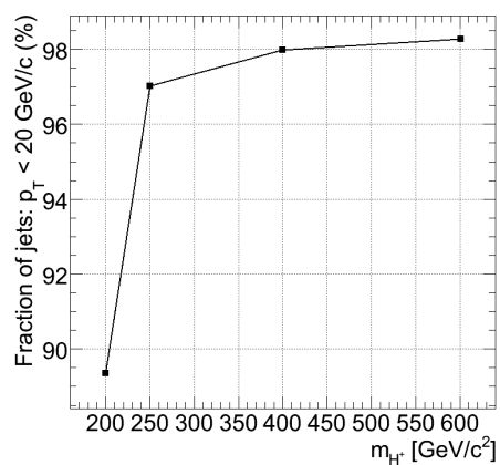
FIG. 6.15 – Fraction de jets de l'événement signal qui passent la coupure sur l'impulsion transverse en fonction de la masse du boson de Higgs chargé.
