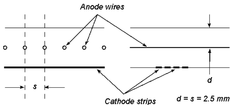
FIG. 2.16 – Schéma d'une station CSC.
