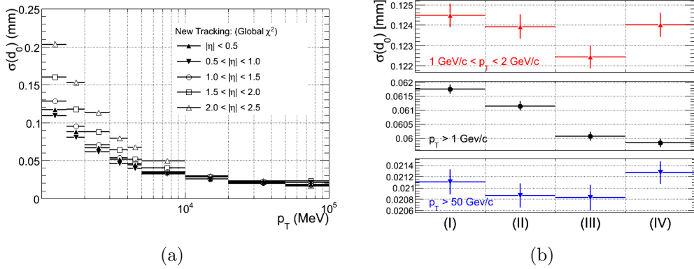
FIG. 4.18 – Résolution du paramètre d’impact transverse : (a) en fonction de l’impulsion transverse et de la pseudorapidité pour les traces reconstruites avec l’algorithme de tracking (I), et (b) en fonction de l’algorithme de tracking utilisé pour plusieurs domaines d’impulsion transverse.
