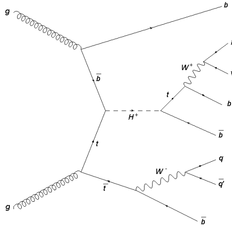
FIG. 5.9 – Un des diagrammes de Feynman possibles illustrant la production et la désintégration d'un boson de Higgs chargé selon le canal étudié.
