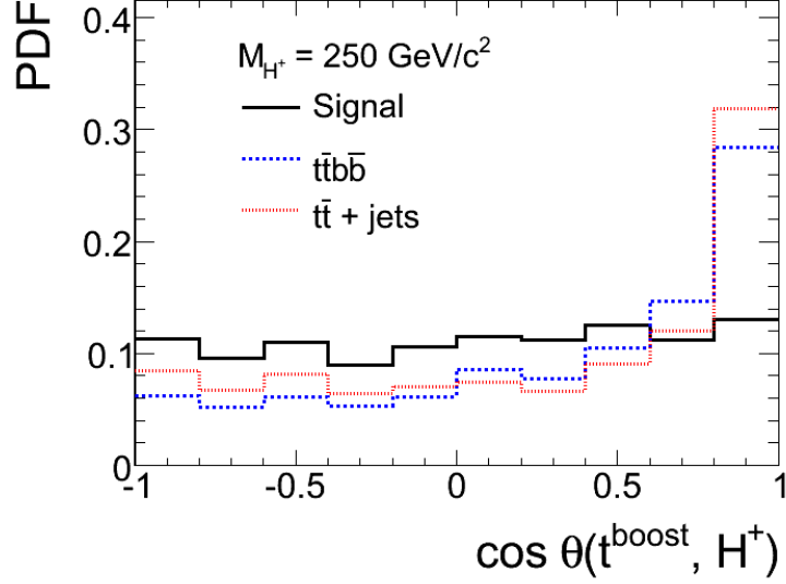
FIG. 6.29 – Distribution de \cos\theta(t^{boost}, H^+) pour les événements de signal (noir) et pour les deux bruits de fond principaux : t\bar{t}b\bar{b} (bleu) et t\bar{t} + jets (rouge), pour les bonnes combinaisons reconstruites en se basant sur la vérité Monte Carlo.
