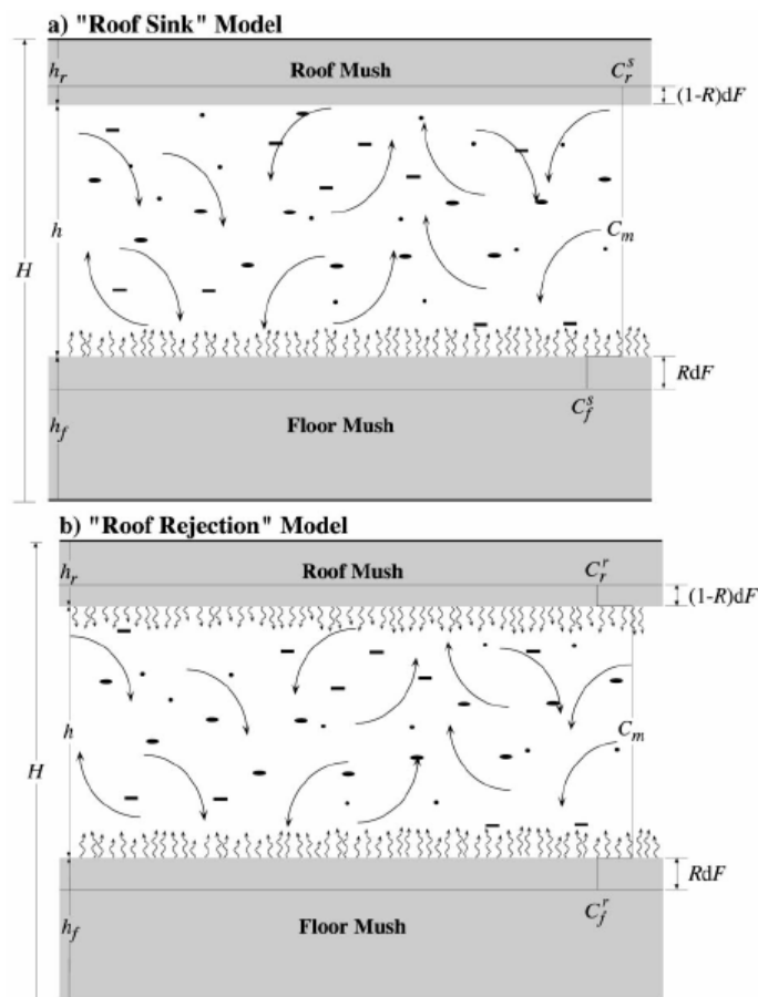
Figure 8 : Schémas descriptifs des modèles de solidification du lac de lave du Kilauea Iki.
