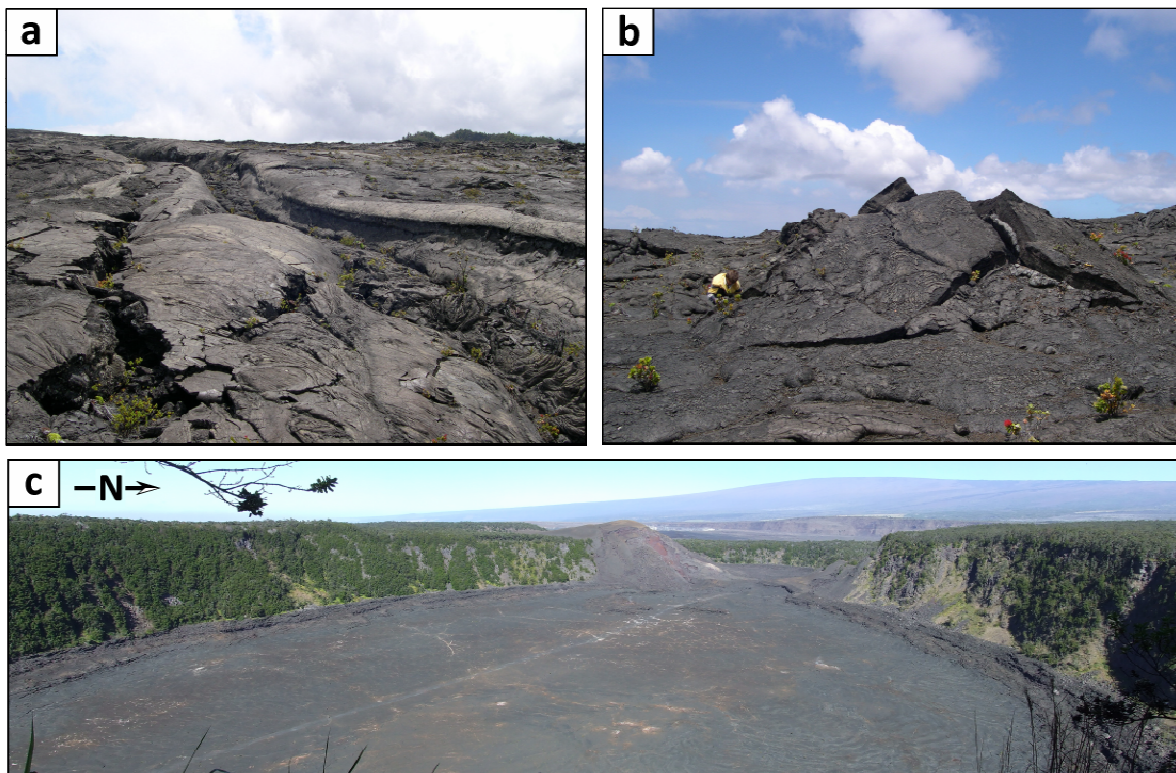
Figure 9 : Photographies des zones étudiées : Mauna Ulu et Kilauea Iki, Hawaii. (a) Champ de lave sur les pentes du Mauna Ulu, mettant en évidence un chenal de lave solidifié ; (b) Échantillonnage d'un bloc de lave au niveau d'un hornito situé dans le champ de lave du Mauna Ulu, proche du cratère Makaopuhi ; (c) Vue d'ensemble du cratère du Kilauea Iki et son lac de lave solidifié, avec en arrière-plan la silhouette du Mauna Loa. Photos prises en Juin 2006.
