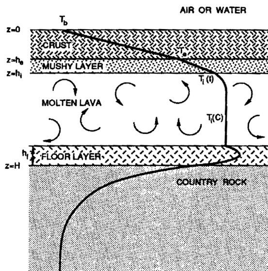
Figure 7 : Modèle simple d'un lac de lave.
