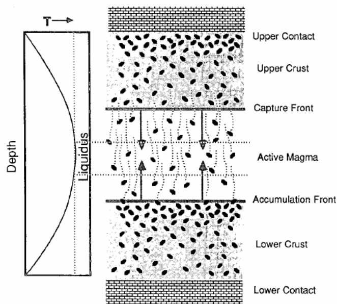
Figure 5 : Colonne de magma schématique.
