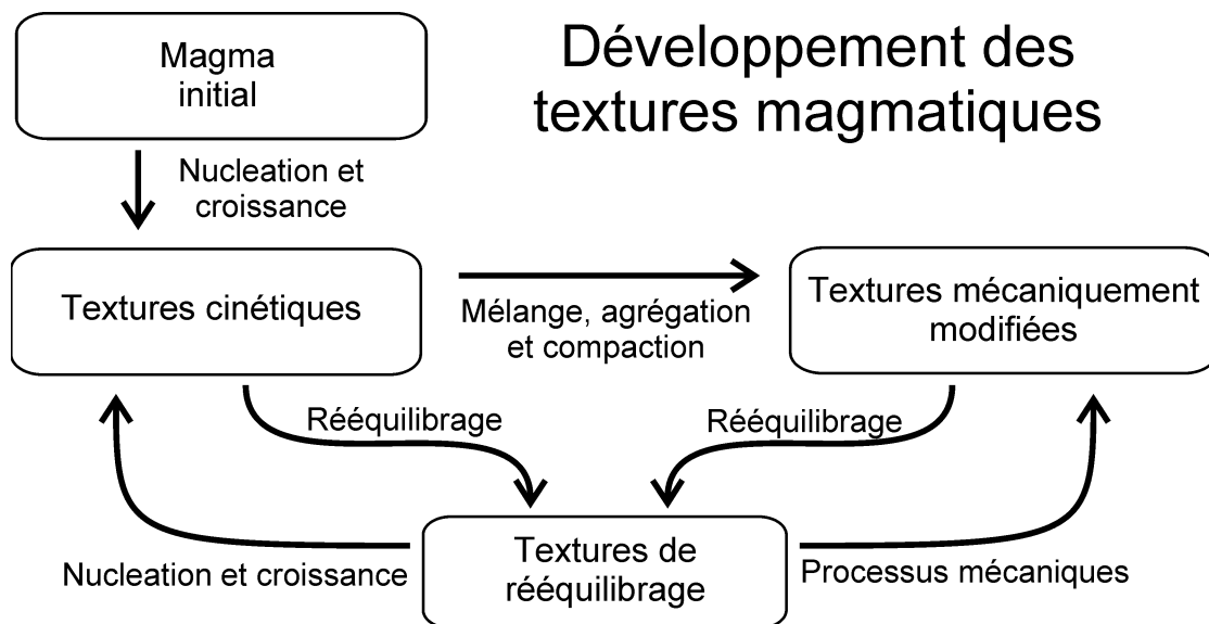
Figure 1 : Développement des textures magmatiques. Rôle des processus cinétiques, mécaniques et de rééquilibrage. Modifiée d'après Higgins (2006)
