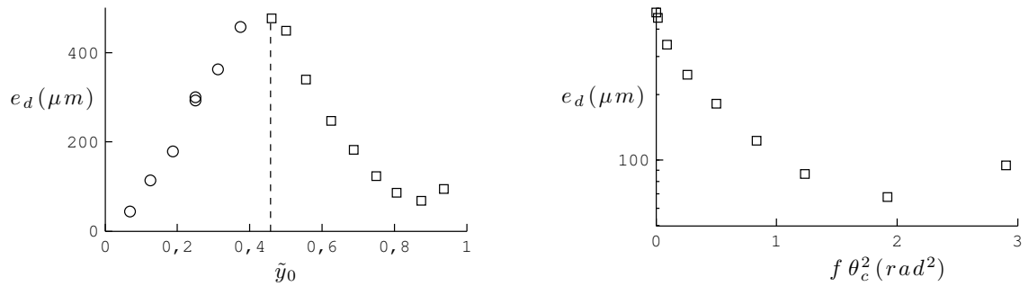
FIGURE 5.6 – À gauche : épaisseur e_d déposée par un racloir flexible en fonction de \tilde{y}_0 . Dans cette expérience, V = 8,2 mm/s, B = 4,2 \cdot 10^{-3} N · m, L = 4 cm et \eta = 17,4 Pa · s. Les pointillés représentent \tilde{y}_0 = \tilde{y}_m . À droite : les données pour y_0 > y_m sont tracées en fonction de f \theta_c^2 (les autres correspondent à \theta_c = 0 ), dans un diagramme semilogarithmique. On n'observe pas la décroissance en \exp(-f \theta_c^2) attendue pour un racloir rigide.
