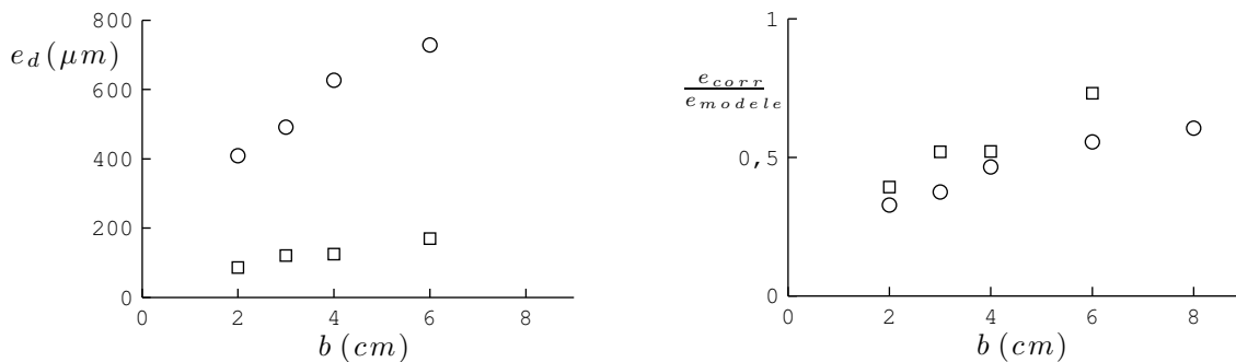
FIGURE 4.18 – Épaisseur de liquide déposé pour différentes largeurs de dépôt b . L = 4 cm ( \circ ) ou L = 2 cm ( \square ), toujours dans la configuration de "mouillage total" ( \tilde{y}_0 = \tilde{y}_m , soit y_0 = 18,4 mm et y_0 = 9,2 mm, respectivement). Les autres paramètres de l'expérience sont \eta = 17,4 Pa·s, V = 8,2 mm/s, B = 4,2 \cdot 10^{-3} N·m. Dans le graphe de droite, l'épaisseur a été corrigée pour tenir compte de la différence entre la largeur de la plaque de dépôt et la largeur du racloir, et adimensionnée par l'épaisseur prédite par le modèle (1,5 mm pour L = 4 cm et 260 \mu\text{m} pour L = 2 cm).
