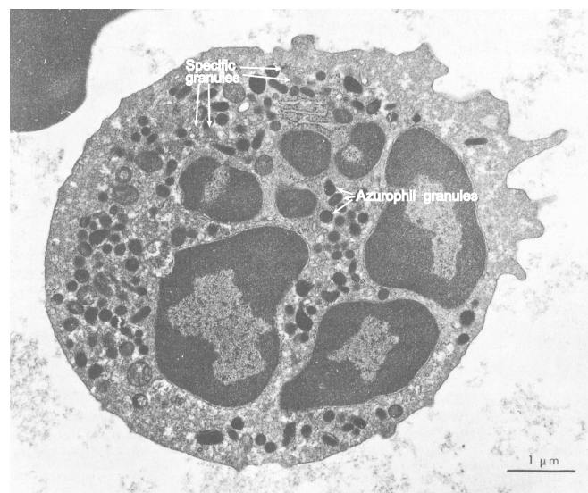
Figure 4: Morphologie d'un leucocyte polynucléaire neutrophile. Leucocyte polynucléaire neutrophile vu en microscopie électronique les lobes nucléaires et les granules cytoplasmiques (azurophiles et spécifiques) sont visibles (Roitt, 1990).
