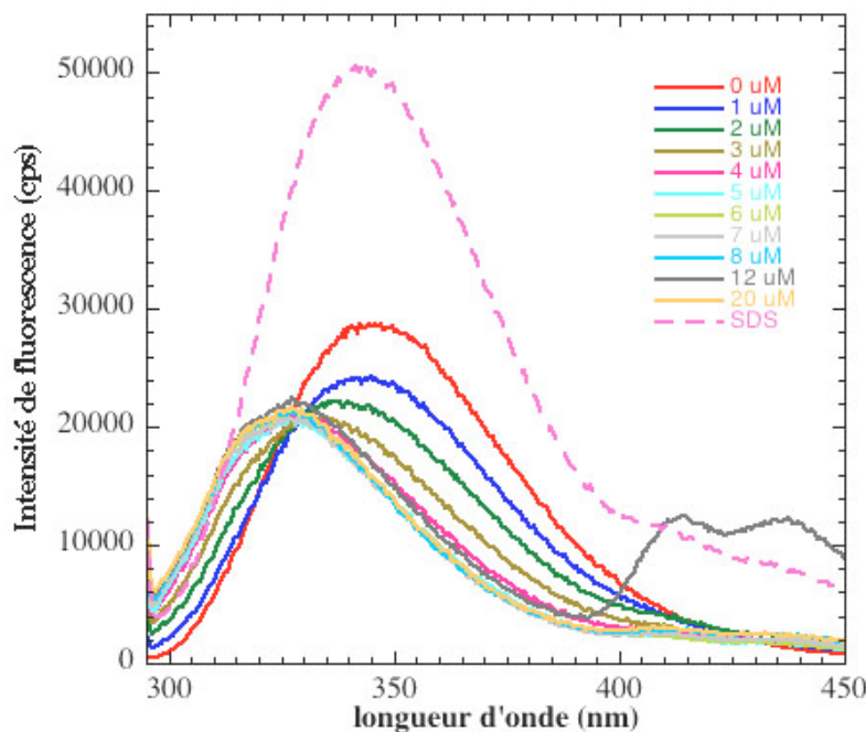
Figure 19 Effet du SDS sur le mélange C-SH3 p67 (5 \mu\text{M} )+peptide « \text{p47}^{\text{phox}} -Cter DDS» (20 \mu\text{M} ). Le spectre en pointillés roses correspond au spectre d'émission de C-SH3 p67 saturé par 20 \mu\text{M} de peptide « \text{p47}^{\text{phox}} -Cter DDS» et en présence de 10 \mu\text{L} de SDS 1%. Les épaulements observés entre 400 et 450 \text{nm} correspondent à la présence d'impuretés dans la cuve expérimentale.
