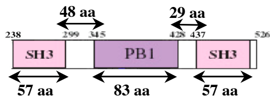
Figure 24 \square Représentation schématique de la région C-terminale de p67 phox . La taille des modules et des régions lien sont indiquées en acides aminés (aa).
