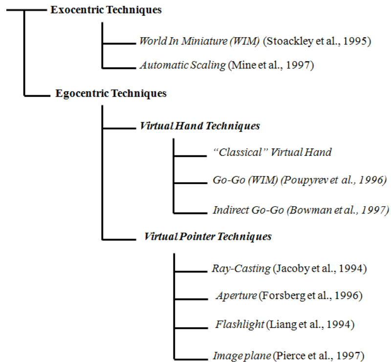
FIG. 2.7 – Classification des techniques de manipulation par métaphore (extrait de [Poupyrev et al. , 1998])
