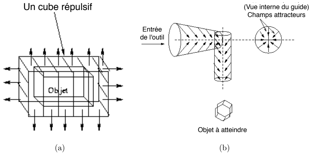
FIG. 4.11 – Exemple de GVs (extraits de [Otmene, 2000]) (a) "répulsif" pour un volume englobant répulsif et (b) "attractif", pour atteindre un objet de l'environnement avec un outil porté par l'avatar.
