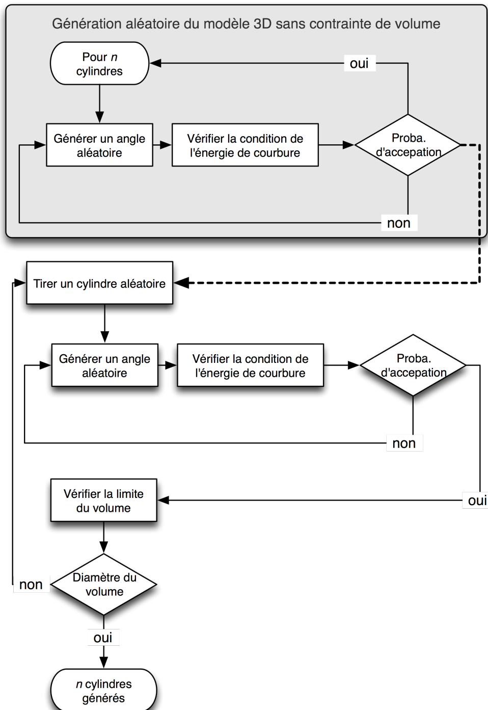
FIG. 3.16 – Le processus de génération des cylindres pour l'algorithme du modèle par compression
