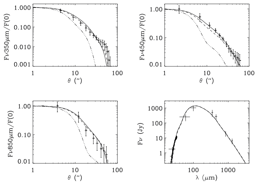
FIGURE 5.4 – Profil d'émission de continu pour la proto-étoile IRAS 16293-2422 à 350 \mu\text{m} (en haut à gauche), à 450 \mu\text{m} (en haut à droite) et 850 \mu\text{m} (en bas à gauche) et la SED entière montrant les contraintes sur la photométrie que le spectre IRS apporte (en bas à droite). Figure tirée de Crimier et al. (2009).
