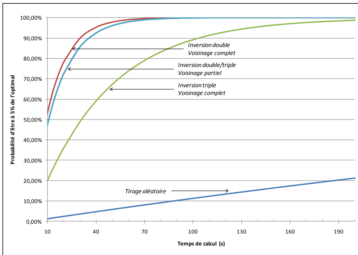
Figure 73 : Performances temporelles de 4 instances de l'heuristique, problème 1
