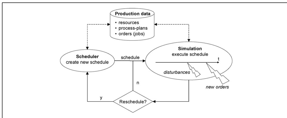
Figure 13 : Architecture d'évaluation d'un ré-ordonnancement
