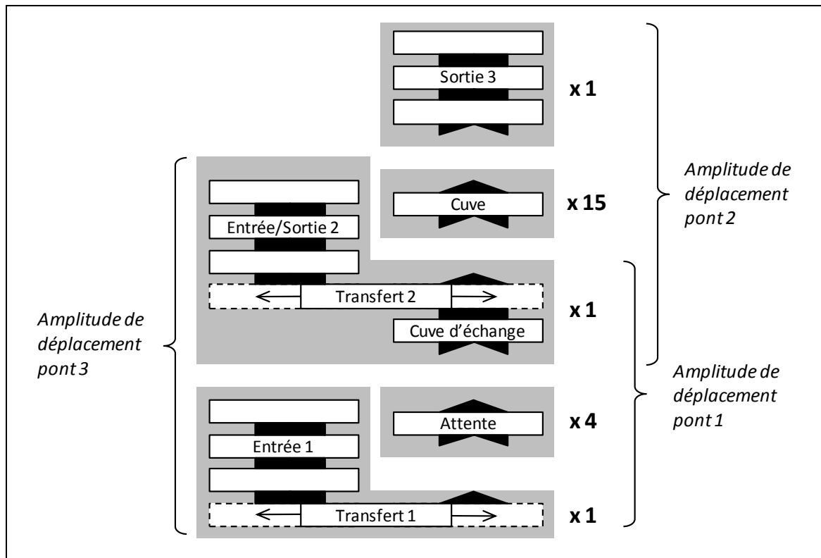
Figure 55 : Blocs élémentaires à implanter pour le cas industriel B
