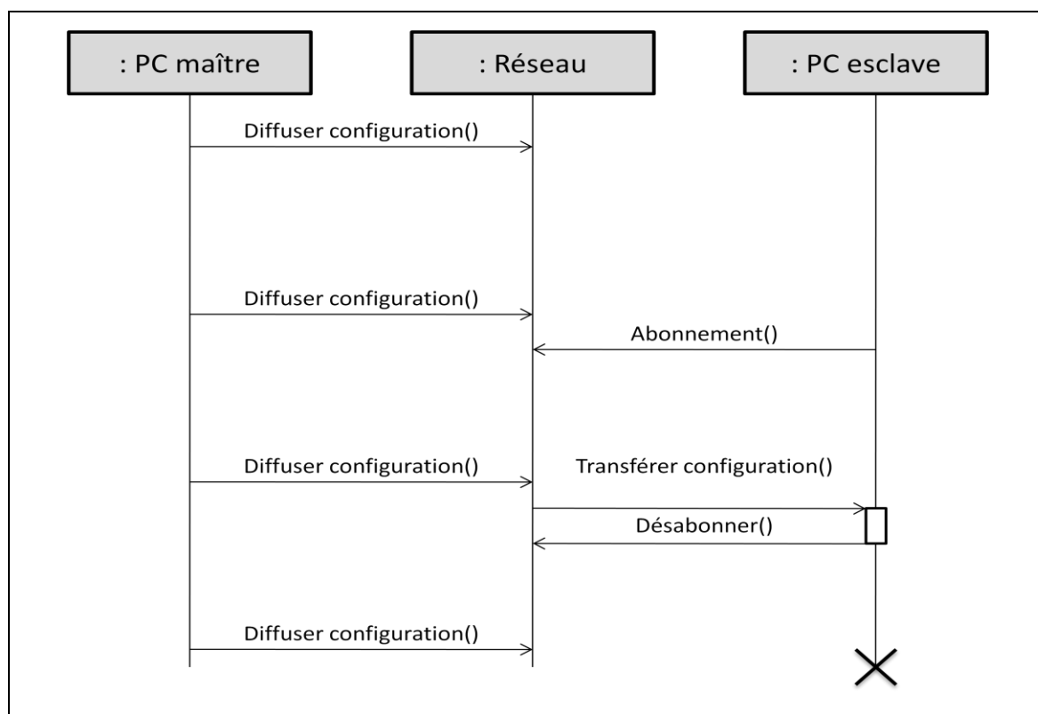
Figure 62 : Protocole d'auto-configuration des esclaves basé sur un flux UDP/IP multicast
