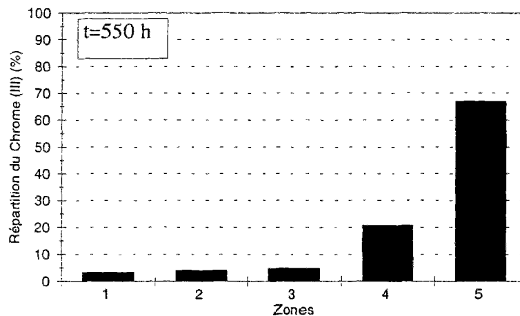
Figures 27 : Répartition du chrome (%) en fonction du temps pour les essais réalisés avec une concentration initiale de 1 g de \text{Cr}^{3+}/\text{l} et pour un champ électrique de 2.6 V/cm (tableaux 6.c-Annexe II)
