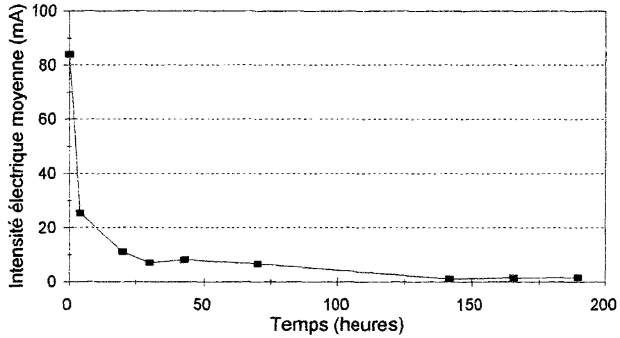
Essais Cr[05]60
