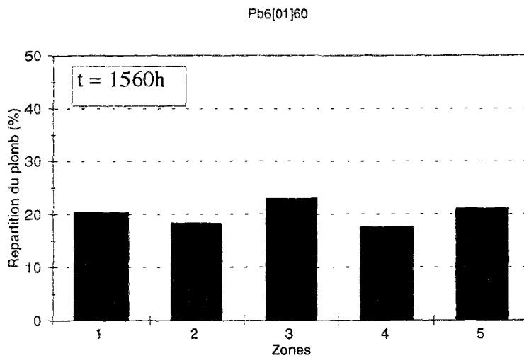
Figures 17 (suite): Répartition du plomb (%) en fonction du temps pour les essais réalisés avec une concentration initiale de 0.1 g de Pb 2+ /l et pour un champ électrique de 2.6 V/cm (tableaux 3.a - Annexe II).
