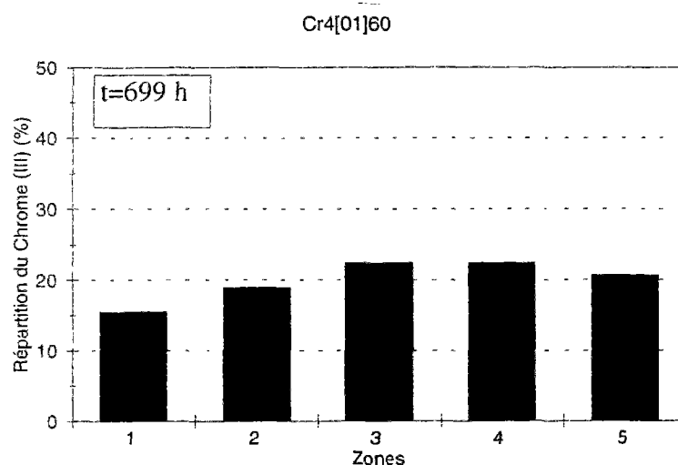
Figures 25 (suite): Répartition du chrome (%) en fonction du temps pour les essais réalisés avec une concentration initiale de 0.1 g de \text{Cr}^{3+}/\text{l} et pour un champ électrique de 2.6 V/cm (tableaux 6.a-Annexe II)
