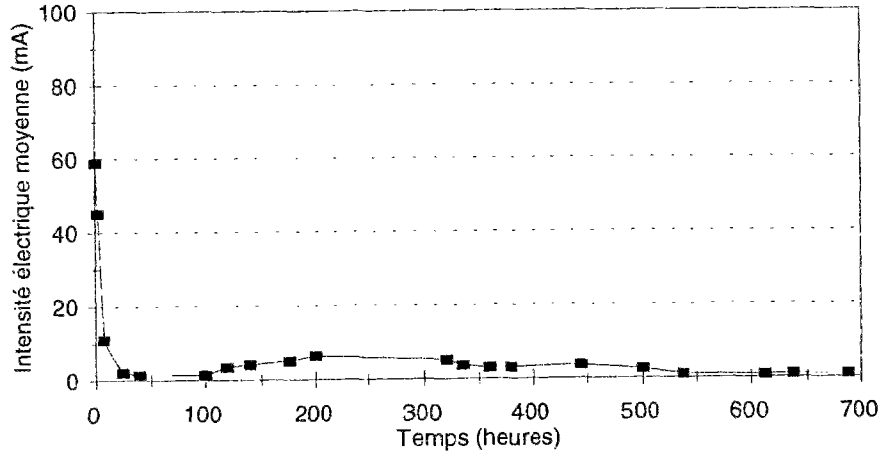
Essais Cr[05]60
