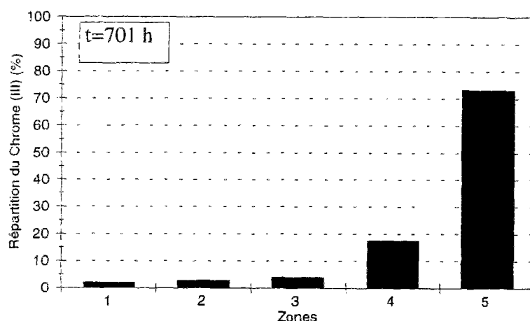
Figures 27 (suite): Répartition du chrome (%) en fonction du temps pour les essais réalisés avec une concentration initiale de 1 g de \text{Cr}^{3+}/\text{l} et pour un champ électrique de 2.6 V/cm (tableaux 6.c-Annexe II)
