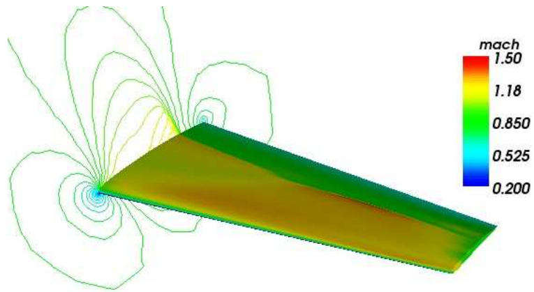
FIGURE 4.18 – Champs et isovaleurs de nombre de Mach : Paramétrisation moyenne ( 6 \times 1 \times 1 )
