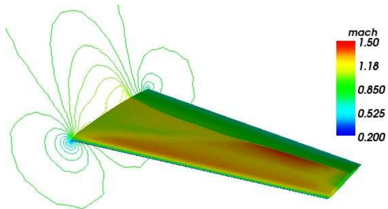
FIGURE 4.19 – Champs et isovaleurs de nombre de Mach : Paramétrisation fine ( 9 \times 1 \times 1 )
