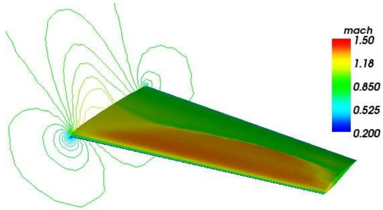
FIGURE 4.17 – Champs et isovaleurs de nombre de Mach : Paramétrisation grossière ( 3 \times 1 \times 1 )
