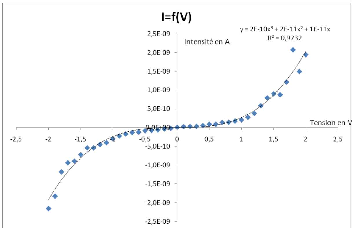
Figure IV.9 : Courbes d'intensité en fonction de la tension d'un nanotube ou fagot métallique (en haut) et d'un nanotube ou fagot semi-conducteur (en bas).
