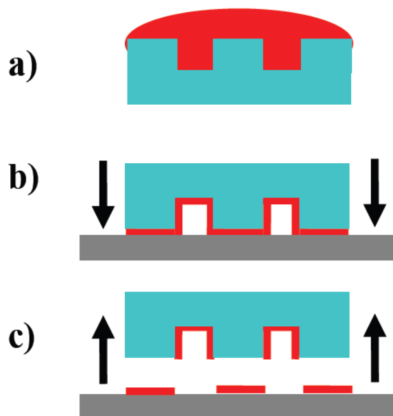
Figure III.25 : Principe du contact printing. a) encrage du timbre : une goutte de solution à transférer est déposée sur la face structurée du timbre. b) Le timbre encré est mis en contact avec le substrat, c) les molécules encrées sur le timbre sont déposées sur le substrat.
