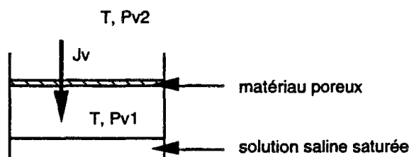
fig. 31 : Illustration de la "méthode de la coupelle".
