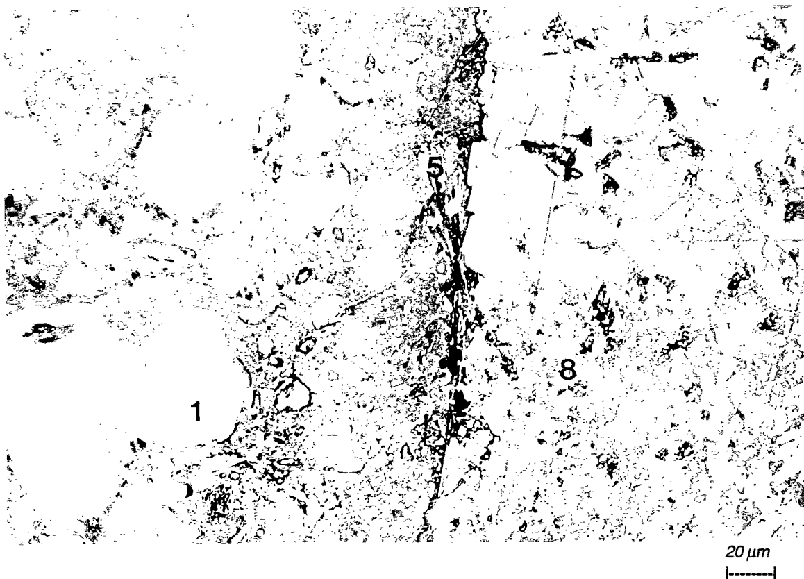
photo 37 : Béton "BH". Interface pâte/granulat calcaire. Faisceaux de \text{Ca(OH)}_2 à l'interface.
