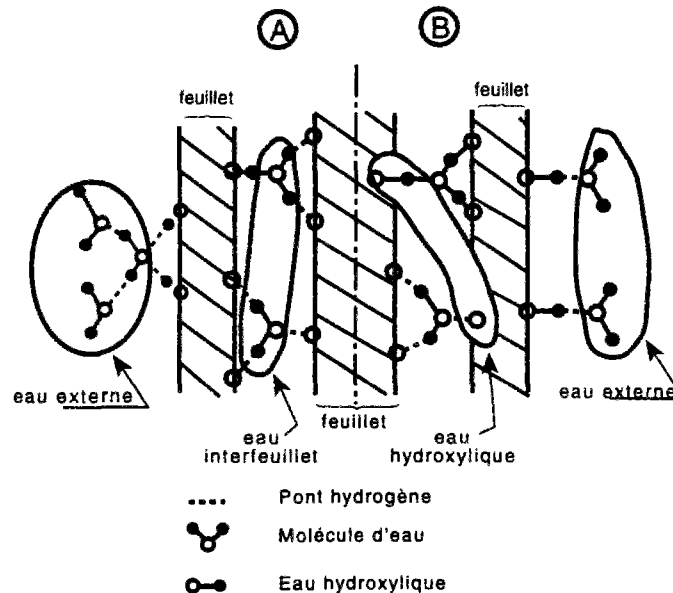
fig. 16 : Schéma illustrant la répartition de l'eau dans l'unité structurale de C-S-H (d'après SIERRA, [20]).
