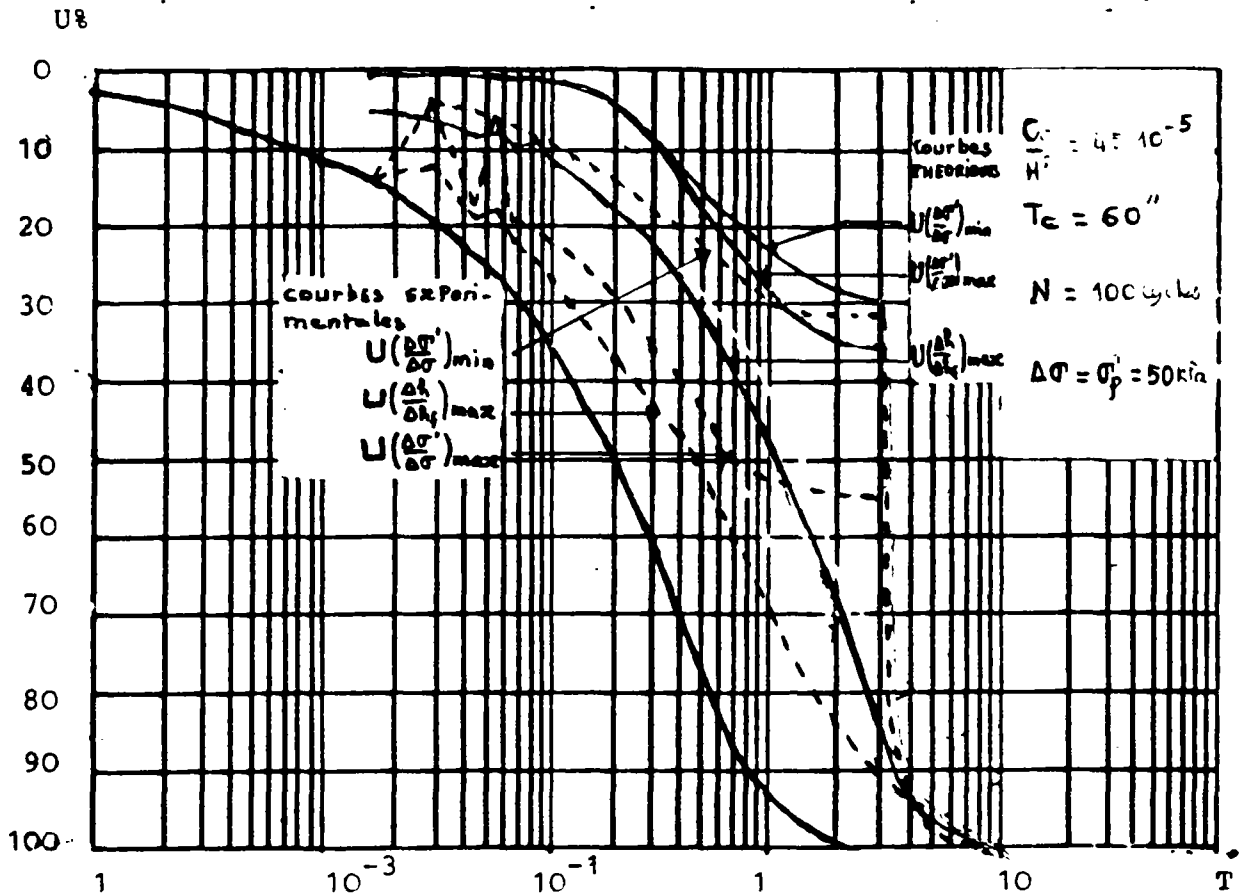
FIG. 70a : Comparaison théorie-expérience à la cellule de Rowe : évolution du degré de consolidation en tassement et en contrainte effective en fonction du facteur temps.
