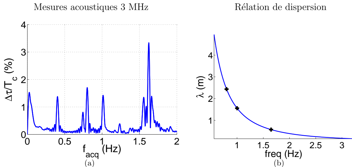
FIG. 3.33 – (a) spectre des PTP, moyenné sur tous les trajets acoustiques. (b) Relation de dispersion des vagues capillogravitationnelles de surface. Les croix indiquent les fréquences et les longueurs d'ondes associées de trois pics de la figure (a)
