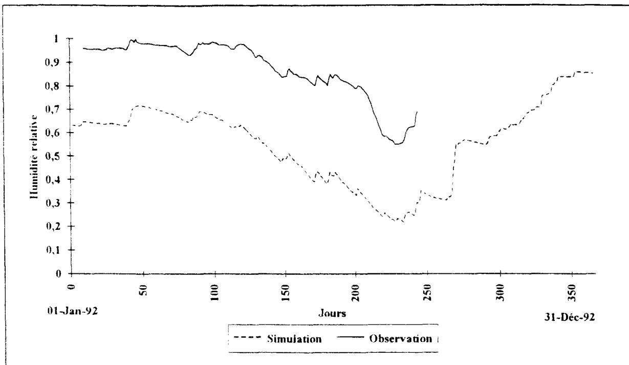
Figure IV-19 : Humidités globales simulées et mesurées à 40 cm.
