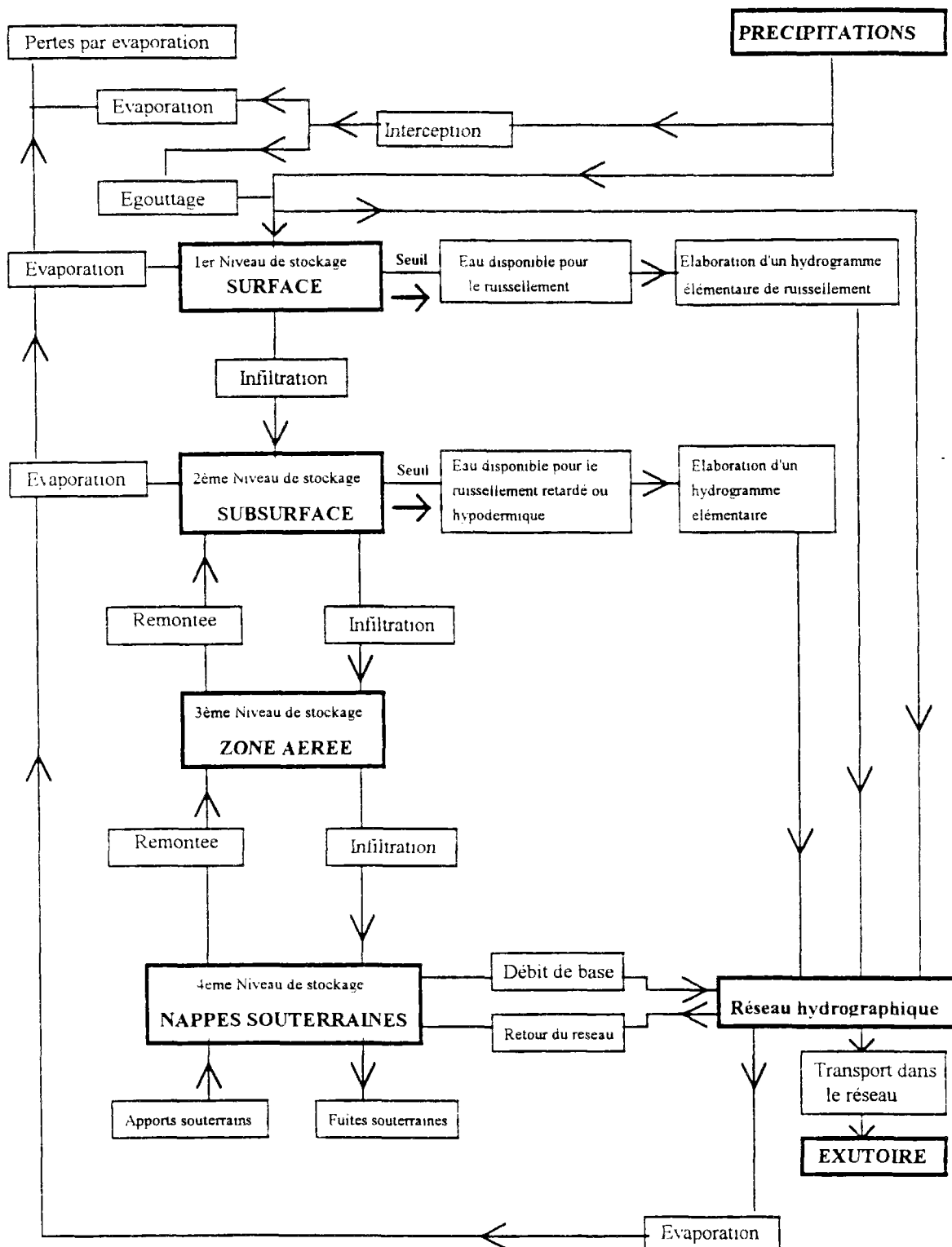
Figure I-1 : Schéma de la phase terrestre du cycle de l'eau (Roche, 1971).
