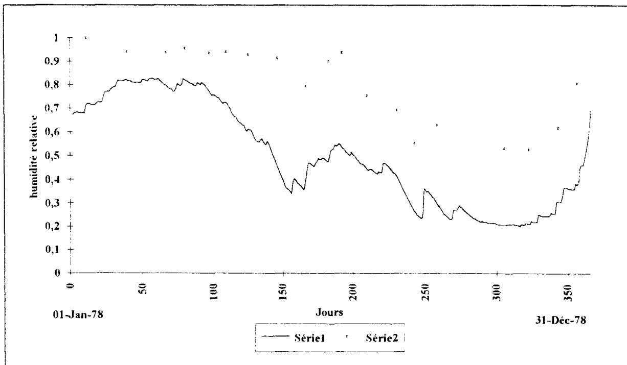
Figure V-11 : Simulation des humidités globales sur l'année 1978.
