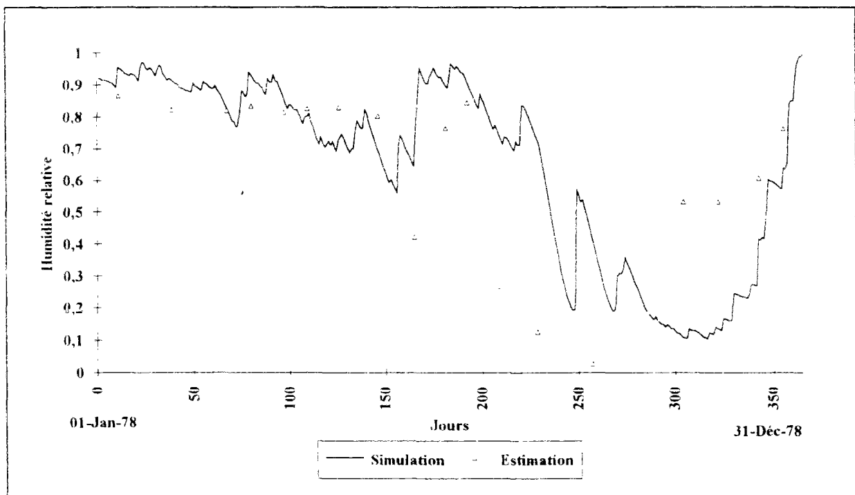
Figure V-12 : Assimilation des humidités de surface sur l'année 1978.
