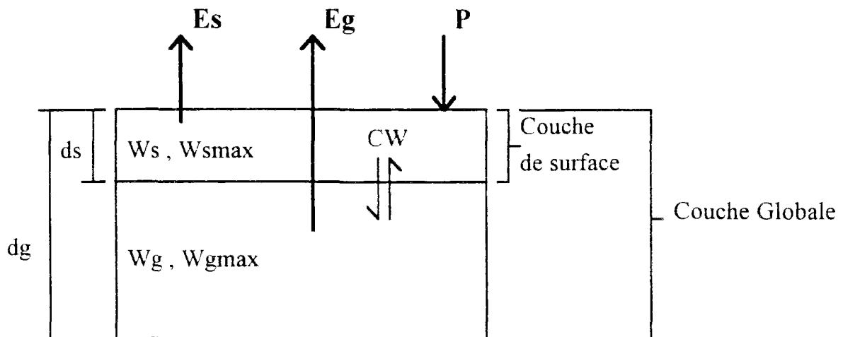
Figure II-7 : Représentation du réservoir-sol par le modèle à deux couches inspiré du schéma de Deardorff (Oulé, 1989).
