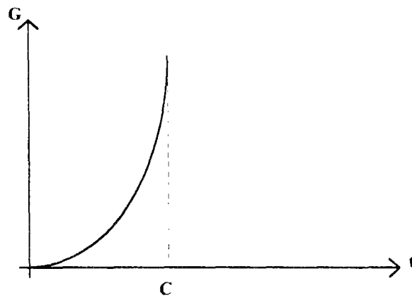
Figure II-2 : Hydrogramme unitaire de l'écoulement "profond".
