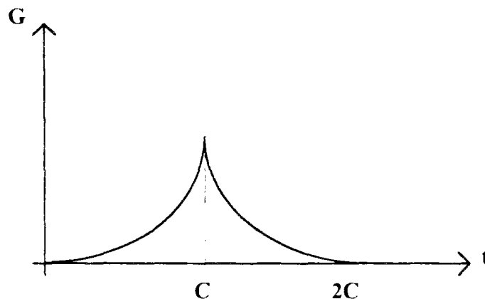
Figure II-3 : Hydrogramme unitaire de l'écoulement "pseudo-direct".
