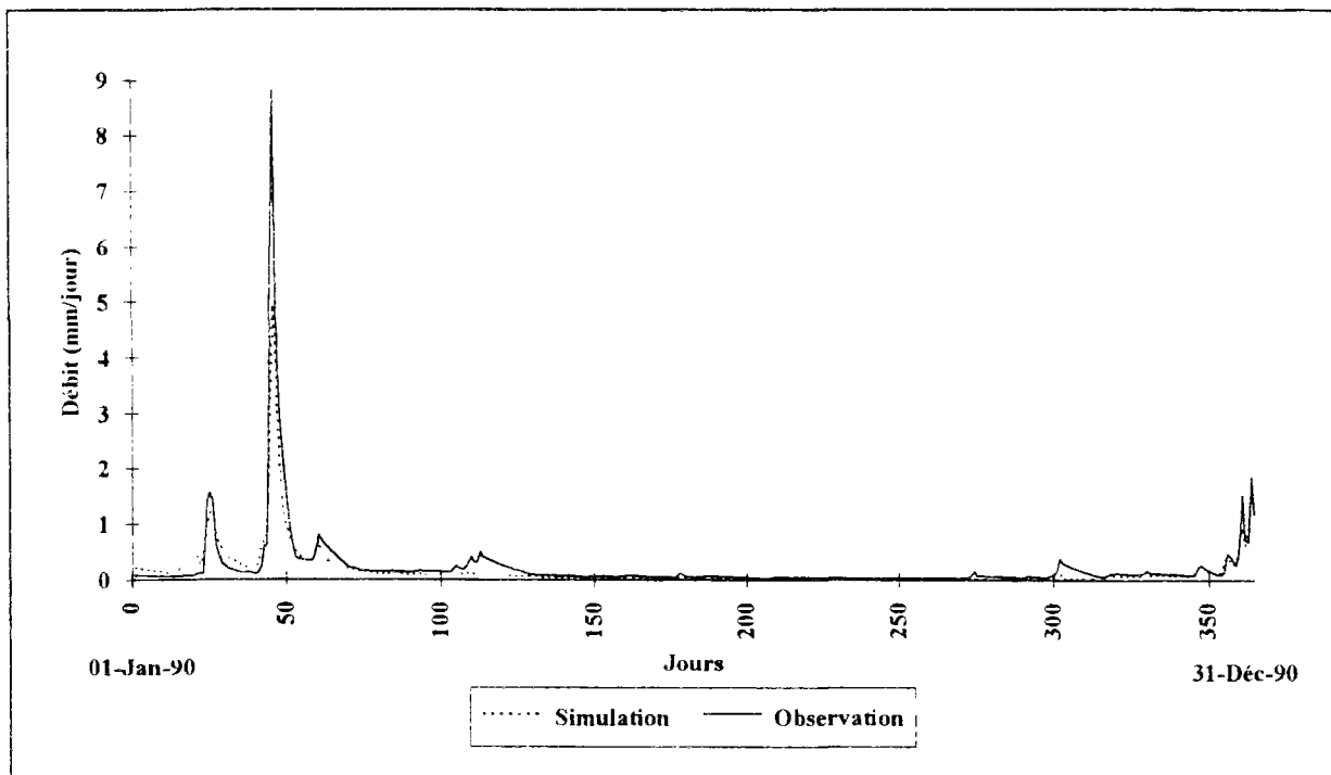
Figure III-6 : Simulation des débits par le schéma de couplage "SHEM4-5". Période de contrôle-Année 1990.
