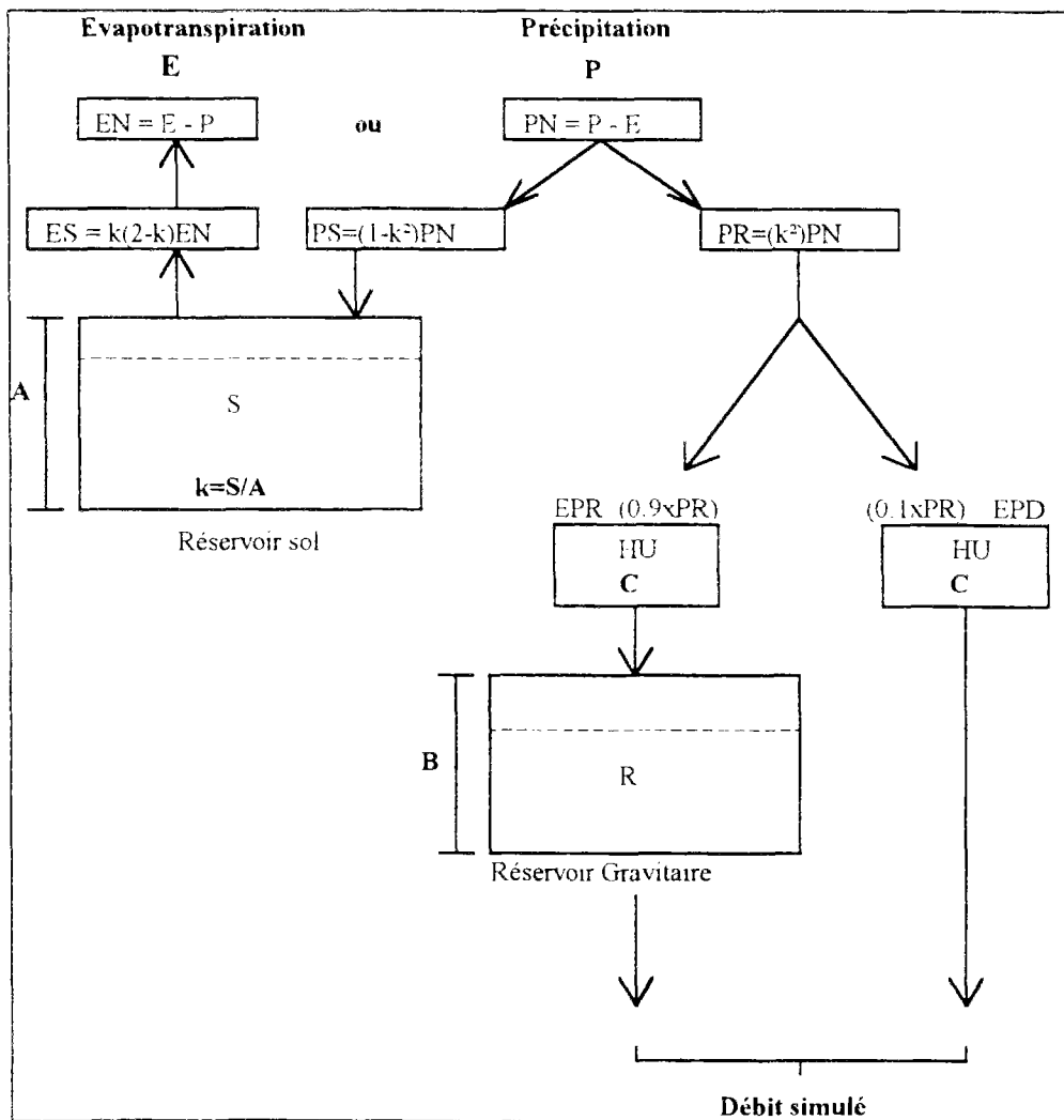
Figure II-1 : Architecture du modèle de base GR3J (Edijatno, 1989).
