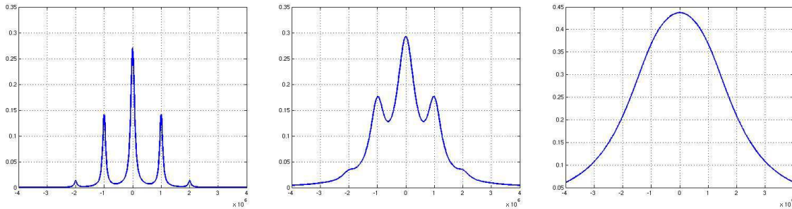
Figure II.5 : Spectre calculé pour un atome à deux niveaux dans le cas d'un mouvement classique caractérisé par k_L X = 1 , \omega/2\pi = 1 MHz. L'excitation laser est caractérisée par une fréquence de Rabi égale à la largeur naturelle : \Omega_L = \Gamma et \Gamma/2\pi = 10^5 Hz (gauche), \Gamma/2\pi = 5 \cdot 10^5 Hz (centre), \Gamma/2\pi = 2 \cdot 10^6 Hz (droit).
