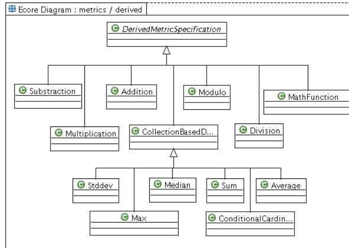
FIG. 3.12 : Opérateurs pour les métriques dérivées
