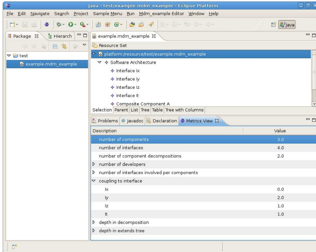
FIG. 3.21 : Outil de mesure généré et intégré dans Eclipse
