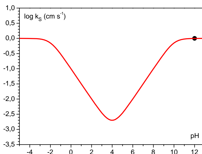
Figure 18 : Variations de la constante de vitesse standard électronique hétérogène en fonction du pH .
