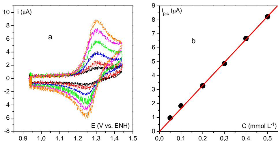
Figure 57 : a. Voltammogrammes du \text{Ru}(\text{bpy})_3^{2+} en milieu aqueux tamponné phosphate ( 0,1 \text{ mol L}^{-1} ), \text{KNO}_3 ( 0,5 \text{ mol L}^{-1} ), \text{pH} = 7 , à différentes concentrations (noir : 0,05 \text{ mmol L}^{-1} , rouge : 0,1 \text{ mmol L}^{-1} , bleu : 0,2 \text{ mmol L}^{-1} , vert : 0,3 \text{ mmol L}^{-1} , rose : 0,4 \text{ mmol L}^{-1} , orange : 0,5 \text{ mmol L}^{-1} ) b. Variation de l'intensité de pic en fonction de la concentration en \text{Ru}(\text{bpy})_3^{2+} dans les mêmes conditions que a (noir : points expérimentaux, rouge : régression linéaire permettant la détermination du coefficient de diffusion D ).
