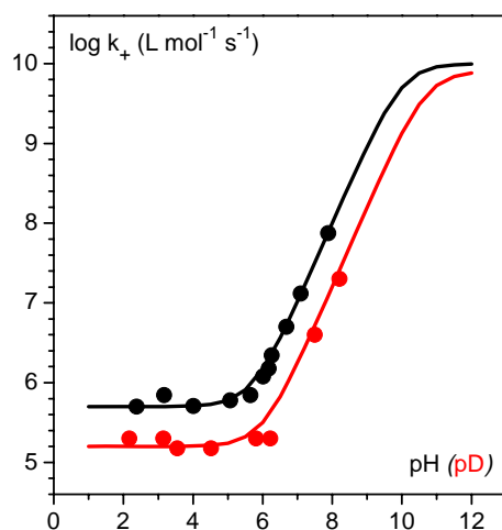
Figure 35 : Variation de la constante de vitesse k_+ en fonction du pH en milieu aqueux non-tamponné protoné (noir) et deutéré (rouge) pour la réaction d'oxydation du phénol par Ru(bpy)_3^{3+} photogénéré. Cercles : expériences, courbes : simulations selon l'équation 24.
