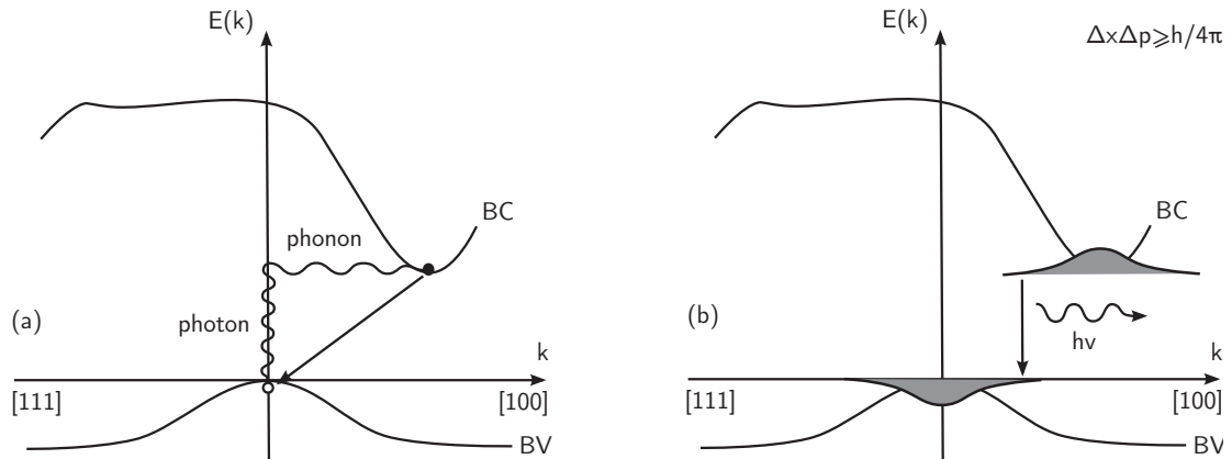
Figure 1.1. Recombinaison de bande à bande dans (a) le Si massif et (b) un nanocristal de Si.
