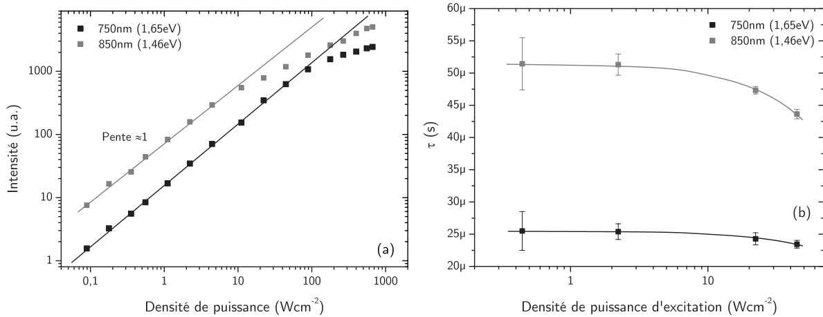
Figure 4.21. Evolution de (a) l'intensité de PL et (b) la durée de vie avec la puissance d'excitation pour deux longueurs d'onde. Même échantillon que celui de la figure 4.20, T=300 K.
