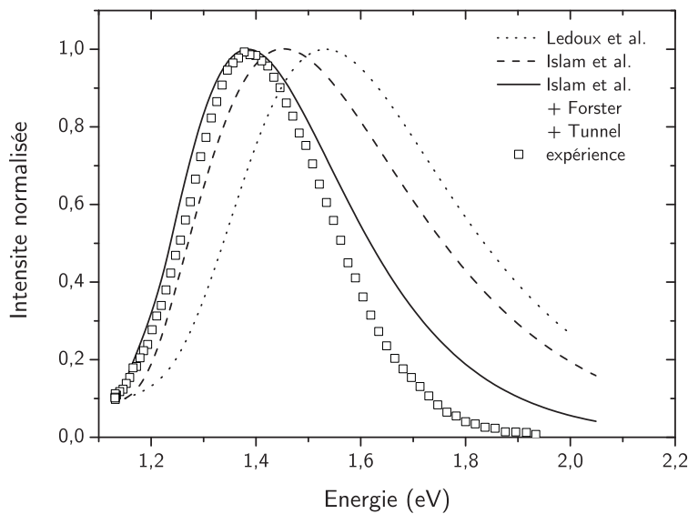
Figure 4.18. Résultats expérimentaux et la modélisation du spectre de photoluminescence par les modèles de Ledoux et al (pointillé) et Islam et al. sans (tirés) et avec (trait plein) les corrections des effets collectifs.
