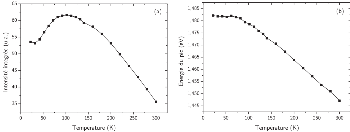
Figure 4.22. Exemple de variation (a) de l'intensité et (b) de la position du pic de photoluminescence en fonction de la température pour un échantillon ayant 11,8% de Si en excès, et recuit suivant RTP 1060°C - 90s + passivation.
