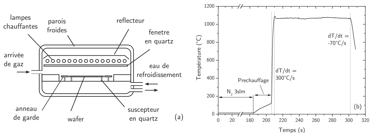
Figure 2.2. (a) Structure du four utilisé pour les recuits rapides et (b) profil type d'un recuit rapide. La rampe de montée est de l'ordre de 300°C/s. La rampe de descente n'est pas contrôlée. Les recuits se font sous atmosphère stagnante de N 2 .
