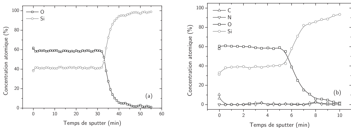
Figure 3.1. Exemple de profil de composition en O (carrés) et Si (ronds) obtenu par XPS pour le procédé à 750°C (a) et à 850°C (b).
