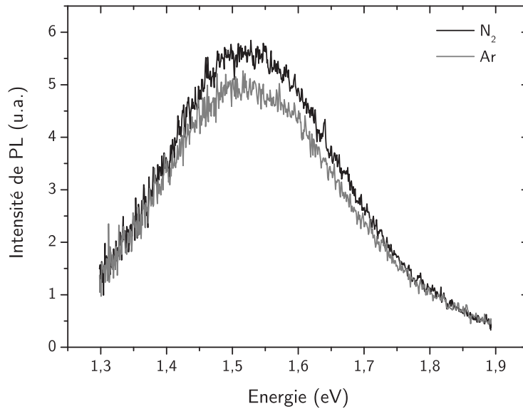
Figure 3.28. Spectres de PL obtenus pour des recuits lents sous Ar (noir) et N_2 (bleu), avant passivation pour un échantillon à 8,5% Si en excès et ayant subi un RTP 1060^\circ\text{C} , 90s + 950^\circ\text{C} - 1h.
