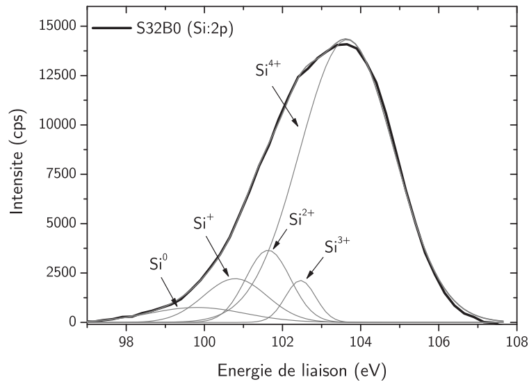
Figure 3.3. Spectre de XPS haute résolution (trait noir) et déconvolution en pics (trait gris fin) correspondant aux différents états d'oxydation du Si pour un échantillon de composition (11,1% Si en excès) voisine de celui de la figure 3.2. Le trait gris épais correspond à la somme des pics.
