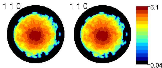
Figure 4 - 26 : Figures de pôles expérimentale et recalculée normalisées, \Delta P_{\{110\}}^{P^-}(\vec{y}, \vec{B}) .
