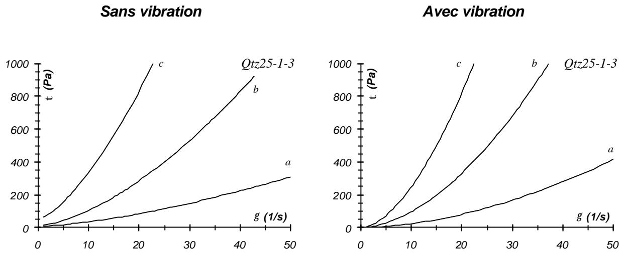
25% quartz broyé avec 3% superplastifiant (SP1)
