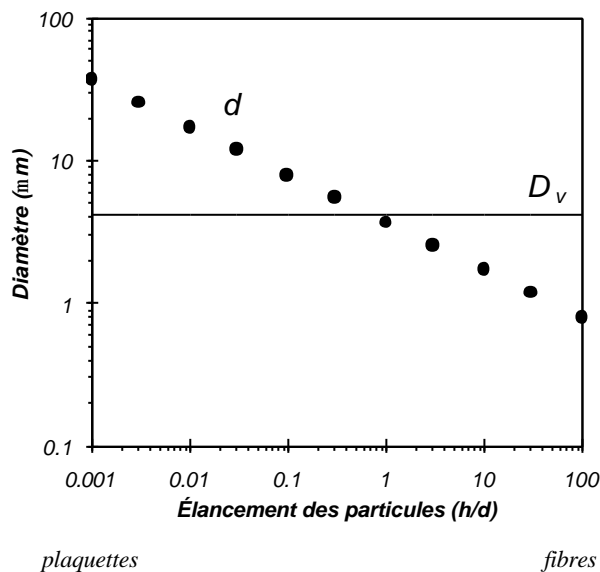
figure 3.10 – Variation du diamètre de particules cylindriques ( d ) d'élongements ( h/d ) variables, ayant le même volume que des sphères équivalentes ( D_v=4,2\mu\text{m} ).
