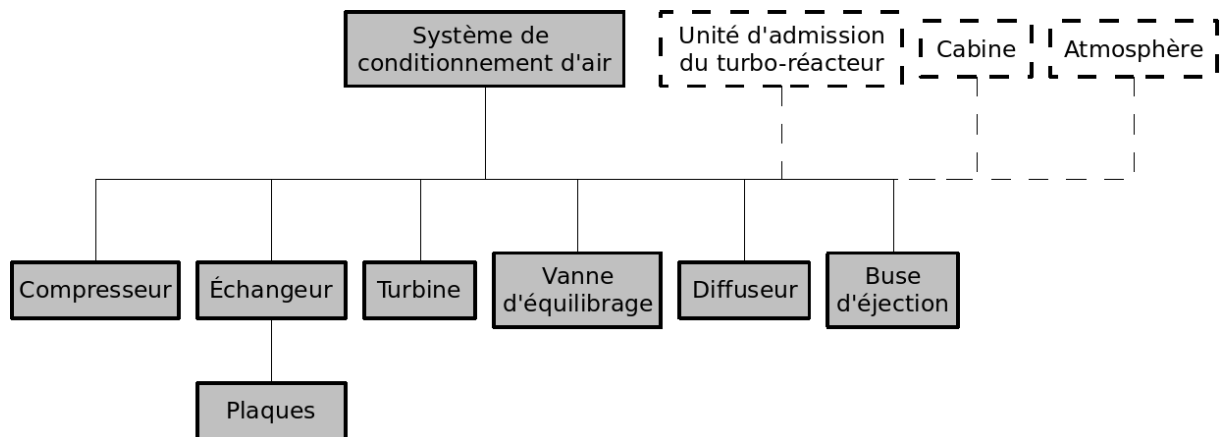
Figure 28 : Organigramme technique étendu du système de conditionnement d'air sans ailette.
