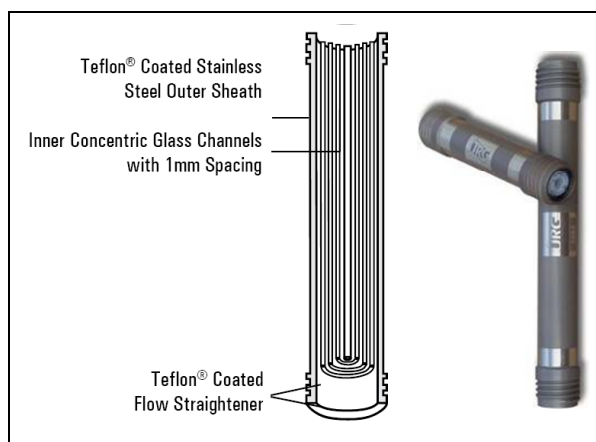
Figure 5 : Coupe interne du denuder URG (modèle 2000-30x150-3CSS).
