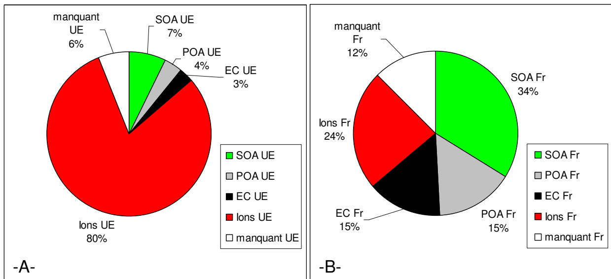
Figure 64 : Composition à Paris de la fraction d'aérosol d'origine continentale (A) et locale (B), Campagne de Paris mai-juin 2007.
