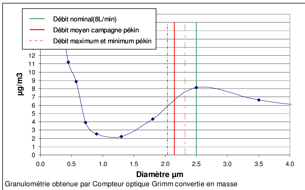
Figure 52 : Granulométrie moyenne obtenue avec l'OPC Grimm, Pékin (aout 2007).
