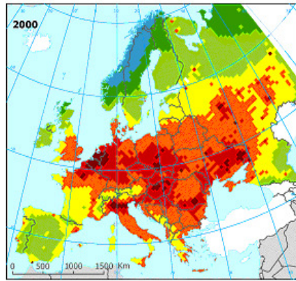
Source : Programme européen CAFE
