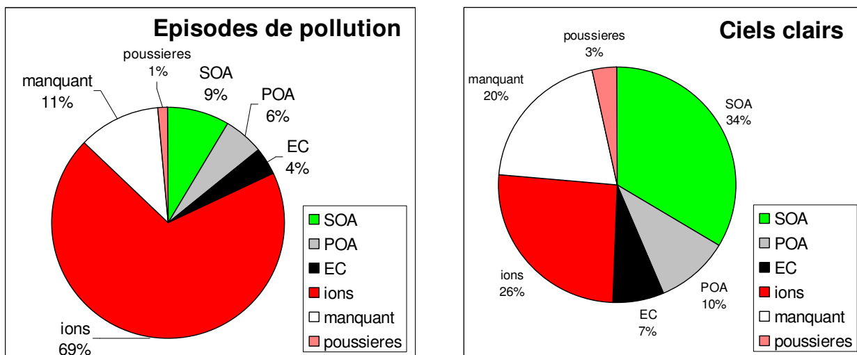
Figure 73 : Composition relative de l'aérosol en cas de pollution et de « ciel clair ».
