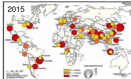
Source : Cartes élaborées par l'Université de Cologne à partir des rapports des Nations Unies
