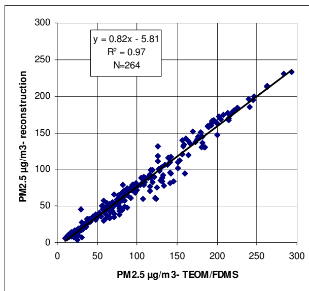
Figure 32 : Comparaison masse TEOM-FDMS & masse reconstruite (chimie rapide).
