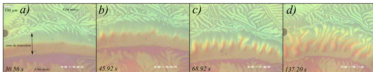
Fig. 6.22: Illustration du processus de digitation observé lors de la coalescence entre deux domaines d'épaisseurs différentes. Sur cet exemple l'épaisseur du film le plus mince est h_1 \approx 230 - 240 \text{ nm} et \lambda_1 \approx 50 - 60 \mu\text{m} tandis que celle du plus épais h_2 \approx 310 - 320 \text{ nm} et \lambda_2 \approx 80 - 85 \mu\text{m} . La taille caractéristique des "doigts" est ici l_{\text{doigts}} \approx 145 \mu\text{m} . Le temps est indiqué en seconde. Le début de la coalescence a eu lieu vers t \approx 0 \text{ s} .
