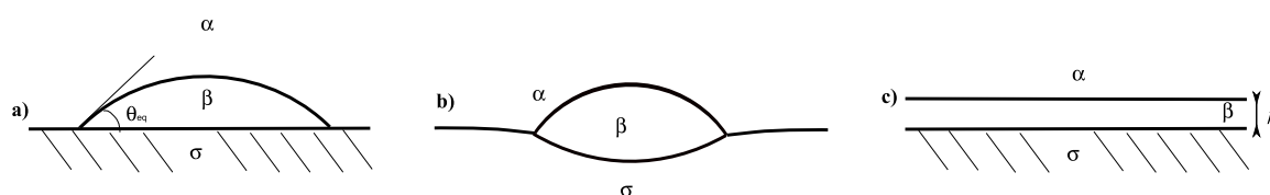
Fig. 1.2: a) Goutte en mouillage partiel sur un substrat solide. b) Lentille de liquide en mouillage partiel sur un substrat liquide. c) Film d'épaisseur h sur une substrat solide.
