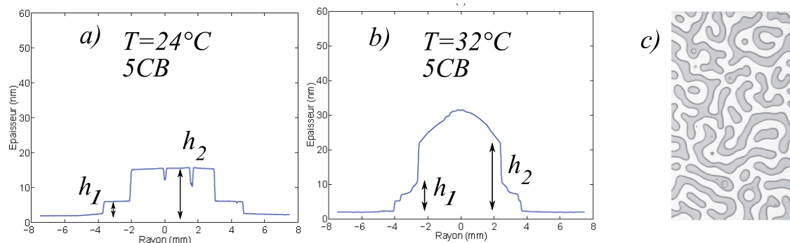
Fig. 2.10: a) Goutte de 5CB à 24^\circ\text{C} sur un wafer de silicium oxydé. b) Goutte de 5CB à 32^\circ\text{C} sur un wafer de silicium oxydé. c) Spin-coating de 5CB sur wafer de silicium oxydé. On observe alors la séparation en deux épaisseurs différentes (D'après [51, 53, 52]).
