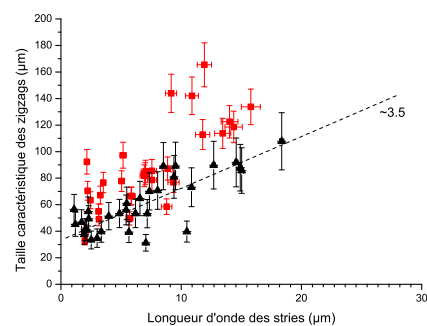
Fig. C.2: Evolution de la taille caractéristique des zigzags en fonction de la longueur d'onde des stries en \mu\text{m} . Deux séries de données effectuées pour le 5CB/Glycérol à température ambiante. La droite en pointillée n'est qu'une aide à la lecture.
