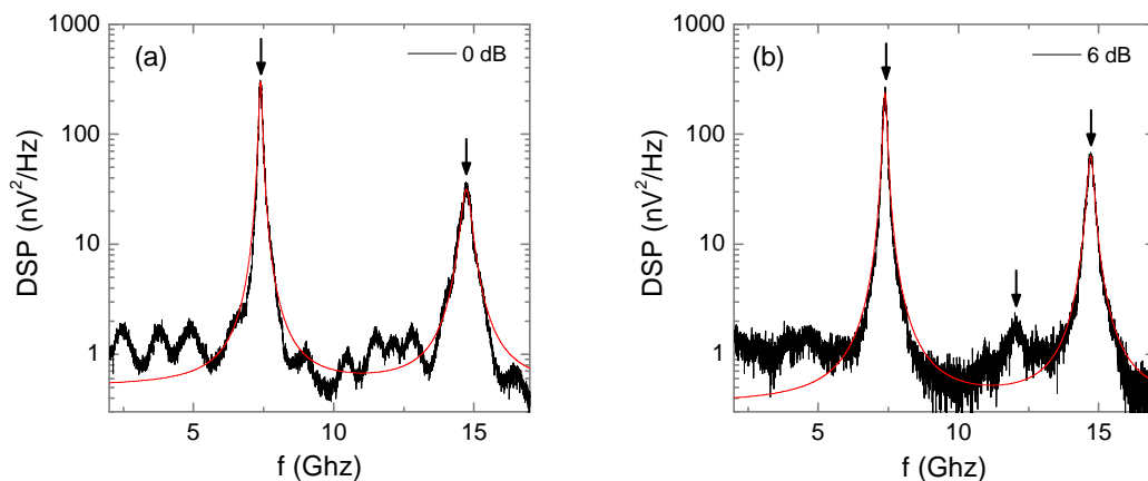
Fig. II.22 – Spectres corrigés de la ligne de base et du gain de la chaîne de mesure pour un oscillateur à jonction tunnel de résistance 530 \Omega . (a) Sans atténuateur. (b) Un atténuateur de 6 \text{ dB} est inséré entre l'échantillon et l'amplificateur. Les flèches noires indiquent les pics identifiés et les courbes rouges sont les ajustements par une Lorentzienne.
