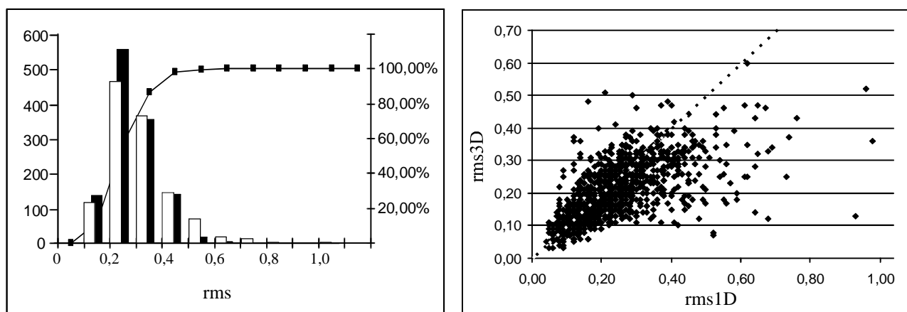
Figure 3.26 - A gauche : histogramme des rms correspondant aux 1208 événements localisés avec les modèles de vitesse 3D et MIN1D (en noir : localisations 3D, m=0,200 s, \sigma=0,087 s; en blanc : localisations MIN1D, m=0,233 s, \sigma=0,122 s). L'amélioration apportée sur les rms par la localisation 3D concerne surtout les rms les plus élevés (entre 0,5 et 1s). Par contre, quelques rms compris entre 0,1 et 0,3 s avec le modèle MIN1D augmentent légèrement avec le modèle 3D comme l'illustre le diagramme des rms3D en fonction des rms1D (à droite, points situés au-dessus de la bissectrice pointillée). Ce diagramme illustre aussi l'amélioration des rms1D supérieurs à 0,5s.
