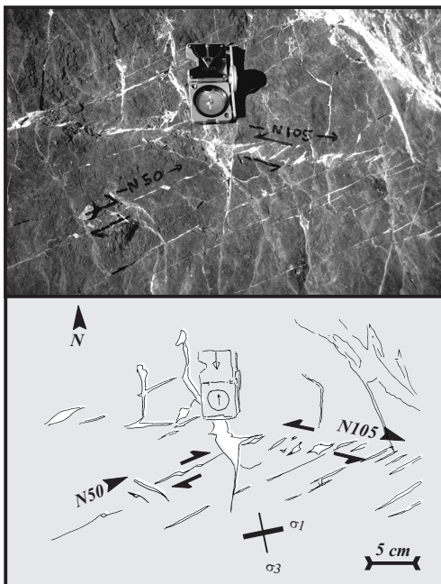
Figure 2.8c : fentes de tension en échelons montrant un cisaillement sénestre selon une direction N105 conjugué avec un cisaillement dextre selon une direction N50 comme en témoignent les micro pull-aparts (entre les deux flèches symbolisant le mouvement dextre). Calcaires du Dogger, site du Pic de Beaudouis.
