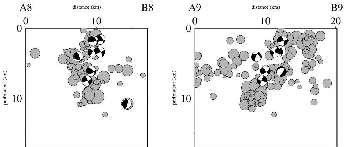
Figure 3.43 - Carte et coupes sismotectoniques de la région de la Haute Ubaye. L'activité sismique et les solutions focales sont, là aussi, bien corrélées avec la fracturation de surface. La coupe A8/B8 est interprétée à la figure 3.44 comme étant en relation avec la faille de Serrenne.
