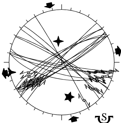
Figure 2.29 - Le site polyphasé de la Croix de la Salcette. Le jeu normal analysé d'un point de vue microtectonique est associé au fonctionnement d'une faille décamétrique parallèle à la faille de la Durance toute proche. Il s'exprime par des failles conjuguées NNW-SSE (longitudinales). Les rejeux décrochants dextres sur cette famille de failles sont associés à des rejeux sénestres suivant les failles ENE-WSW (famille transverse) qui font office de décrochements conjugués.
