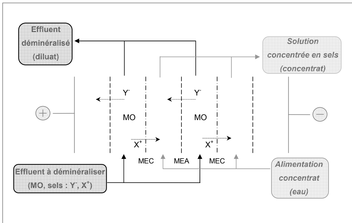
Figure I-2 : Schéma de principe – Electrolyse conventionnelle à deux compartiments
