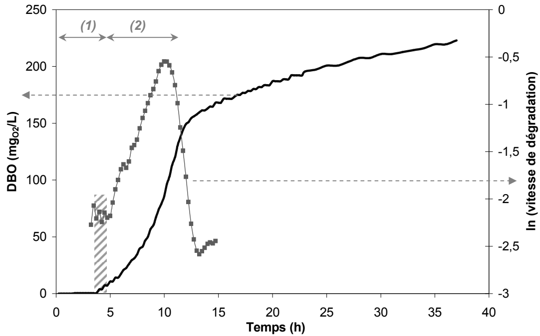
Figure IV-1 : Exemple de détermination du taux de croissance et du temps de latence. [\text{NaAc}] = 0,002 \text{ mol.L}^{-1} et [\text{NaCl}] = 0,16 \text{ mol.L}^{-1} . (1) : Zone d'acclimatation, (2) : Zone de croissance
