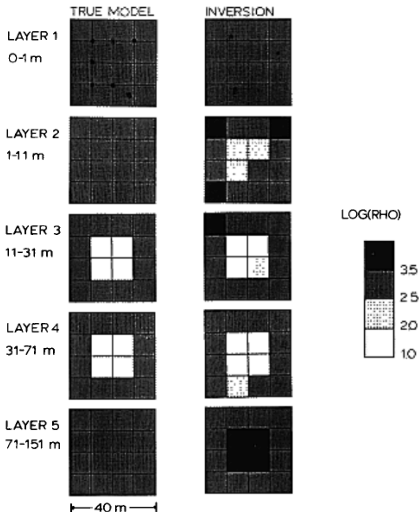
FIG. 2.2: Comparaison du résultat de l'inversion 3D et du modèle synthétique qui a permis de générer les données. Le modèle synthétique est constitué d'un conducteur de 10 Ohm.m plongé dans un résistant de 1000 Ohm.m. L'échelle de couleur est en logarithme (base 10) et les points noirs sur la couche 1 du modèle synthétique représentent les points sources d'injections (7 sources) (d'après Park and Van (1991)).
