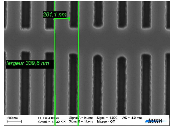
(b) d = 1 \mu\text{m} pas visé : 350 nm, pas obtenu : 340 nm
