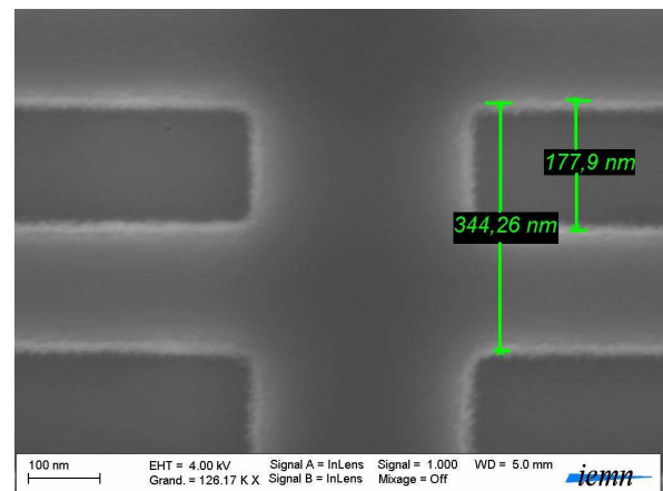
(c) d = 5 \mu\text{m} pas visé : 350 nm, pas obtenu : 344 nm
