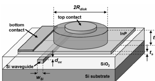
(c) laser à base de microdisque en filière InP couplé à un nanofil en filière SOI [16]
